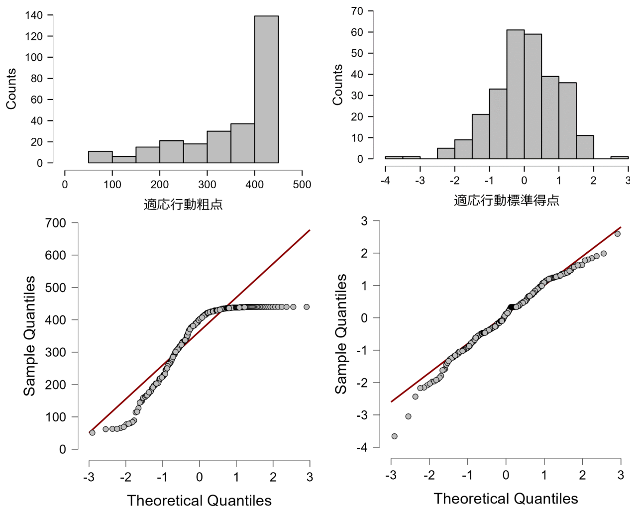
Figure 12 定型発達群における適応行動の粗点 (左列) および標準得点 (右列) のヒストグラム (上段) および Q-Q プロット (下段)
