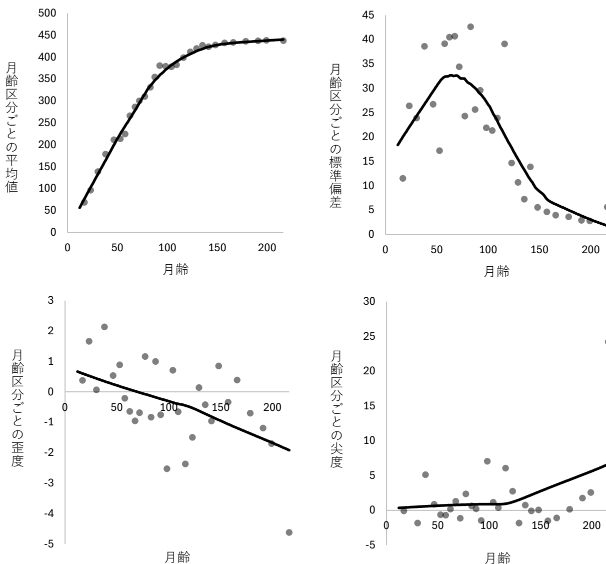
Figure 11 定型発達群における月齢区分ごとの適応行動尺度の粗点の平均値(左上)、標準偏差(右上)、歪度(左下)、尖度(右下)
