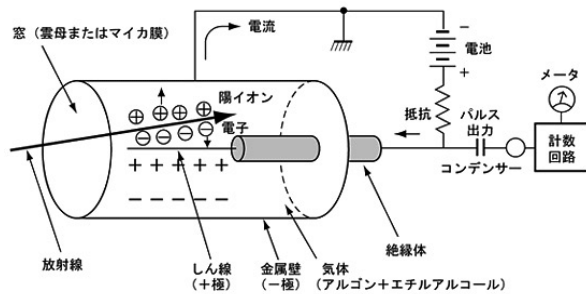
（上図）GM 計数管の原理
