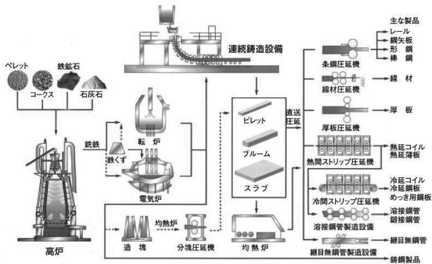
【図表 2-3-1：電気炉・高炉による製鋼法】
