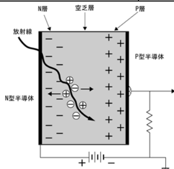
（上図）半導体検出器の原理
