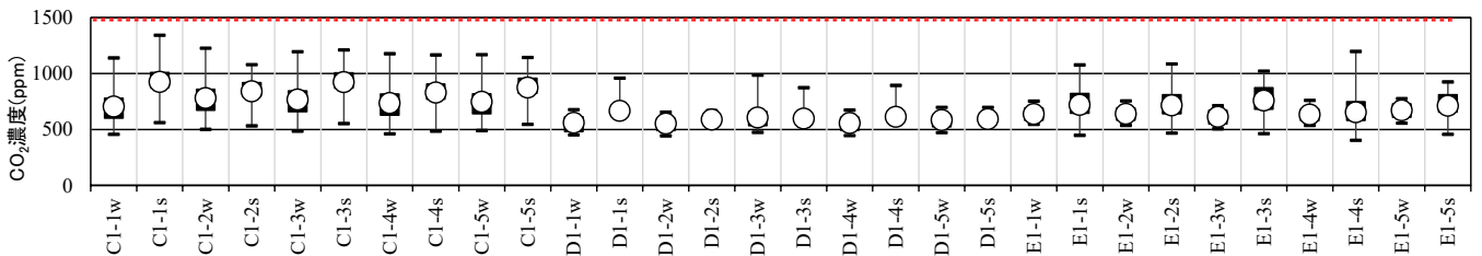
図3 観覧場の二酸化炭素濃度分布 注1), 注2) (施設 C~E, 開演時間~終演時間まで, OA:外気)
