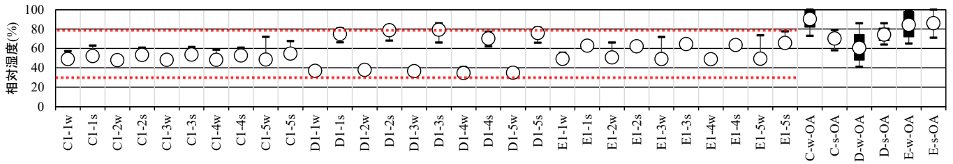
図2 観覧場の相対湿度分布 注1), 注2) (施設 C~E, 開演時間~終演時間まで, OA:外気)
