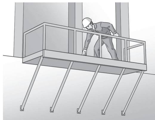
【張り出し足場 22 】
