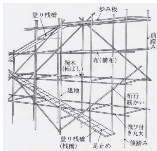
(入りさん橋の図)
