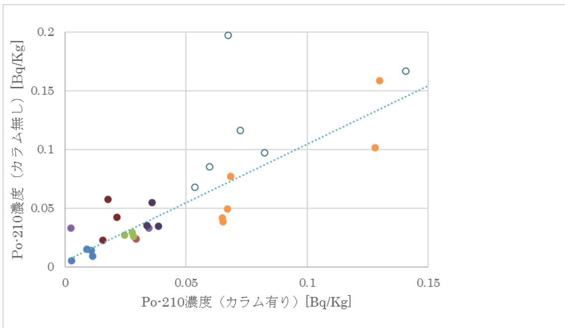
図3 キレート抽出カラムの有無によるポロニウム 210 の測定値への影響
