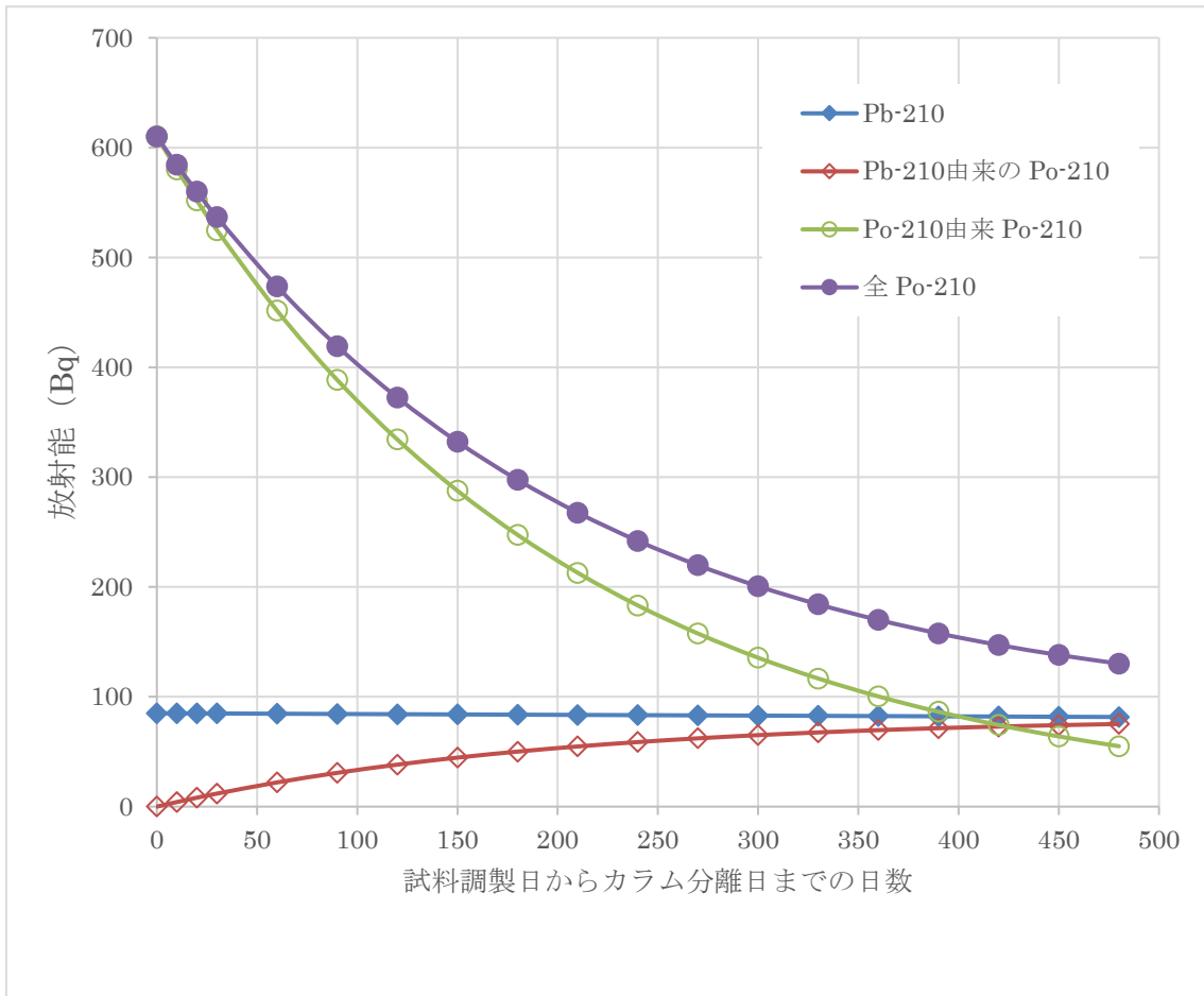
図6 試料調製日からの経過日数による Po-210 および Pb-210 の放射能の経時変化 試料調製日の放射能を Po-210 : 610 Bq、Pb-210 : 85 Bq とした場合の、試料調製日 からカラム分離日までの経過日数による、放射能の経時変化
