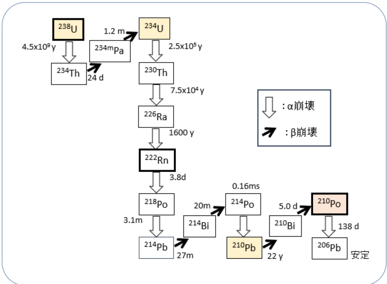
図2 ウラン壊変系列図
