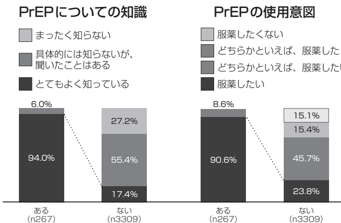
図 2.7 過去6ヶ月間のPrEP服用経験別知識と使用意図
