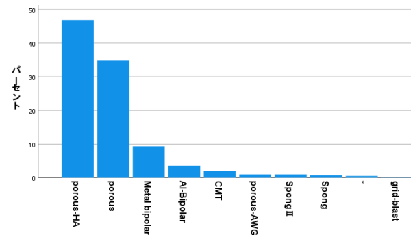
図5. 股臼部品の外表面仕上げ: グラフは左から HA 添加 porous coating 47%、porous coating 35%、金属BP9%、アルミナBP4%など。
