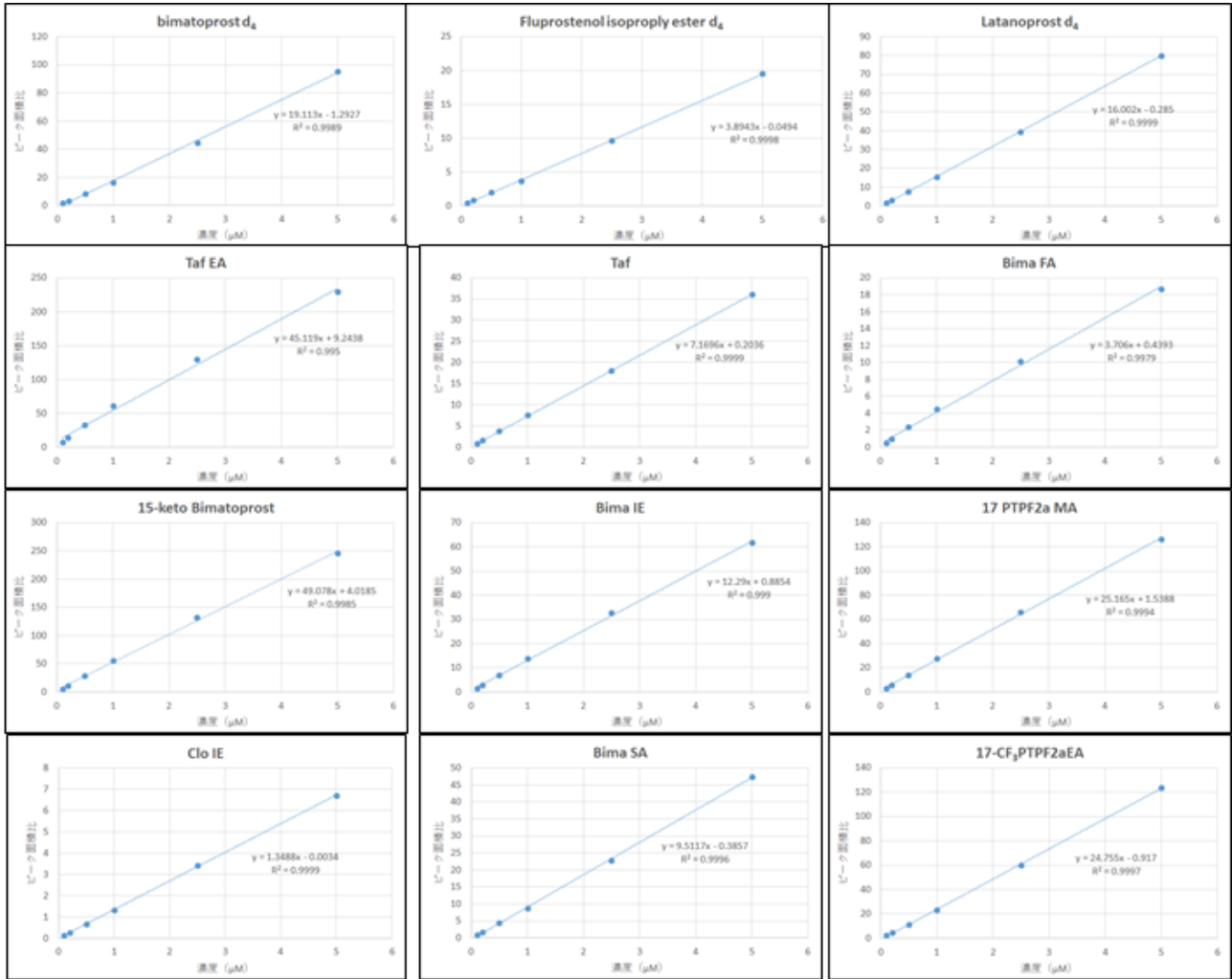
図3 内部標準法による各標準物質の検量線
