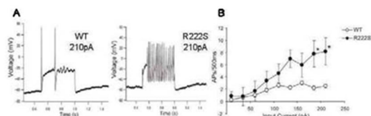
図2: SCN11A p.R222S 変異を持つマウスの神経活動 疼痛経路の DRG ニューロンの発火活動を解析した。野生型 (WT) に比べ、Nav1.9 変異型 (p.R222S) では、同じ入力刺激に対して発火電位の発火が容易になっている (A)、入力刺激 (機械) に対する発火電位の数 (膜電位) を示す。変異型では入力刺激に比例して、発火電位の数が増加し (B)、疼痛経路が活性化されていることを示す。(参考文献 1)より改変)
