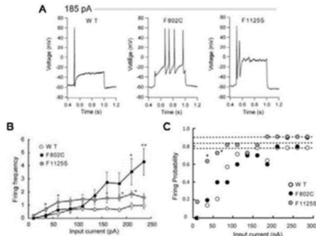
図3: SCN11A p.F802C, p.F1146S 変異を持つマウスの神経活動 SCN11A p.F814C, p.F1146S 変異の相同遺伝子変異 (p.F802C, p.F1125S) を持つ変異型マウスの発火活動を示す。p.F802C 変異型マウスでは p.R222S と同様発火頻度が上昇している (A, B)。一方、p.F1125S 変異型マウスでは小さな入力に対する応答性 (発火に至る確率) が高くなっていることを示す (C)。(参考文献 3) より
