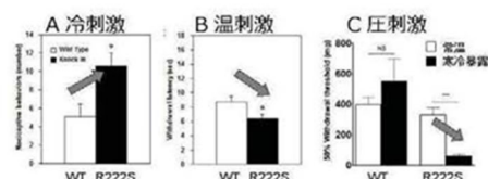
図1: 小児四肢疼痛発作症モデルマウスによる疼痛行動変異 野生型 (WT) に比べ、Nav1.9 変異型 (p.R222S) のマウスは冷、熱刺激に対する痛みの感じやすさが増大している (A, B)。また寒冷暴露条件によって機械刺激に対する疼痛閾値の低下を示し (C)、モデルマウスにおいても小児四肢疼痛発作症の特徴の一つである寒冷により痛みを感じやすくなる性質を持つことを示している。(参考文献 1)、2)より改変)
