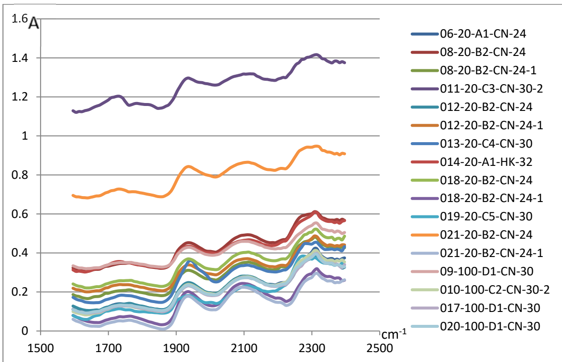
図 6-4 NIR の結果 (4) 100mg 模造品と 20mg 模造品の比較
