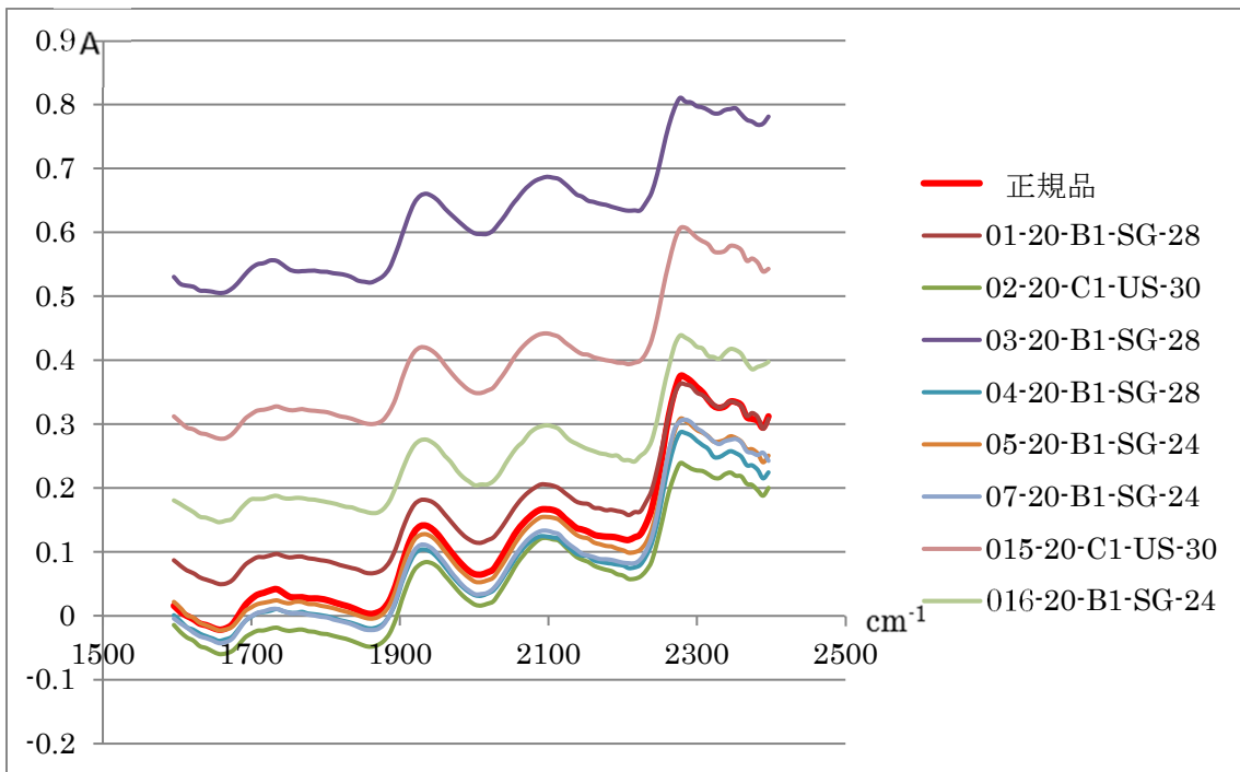
図 6-1 NIR の結果 (1) 20mg 真正品と 20mg 正規品の比較
