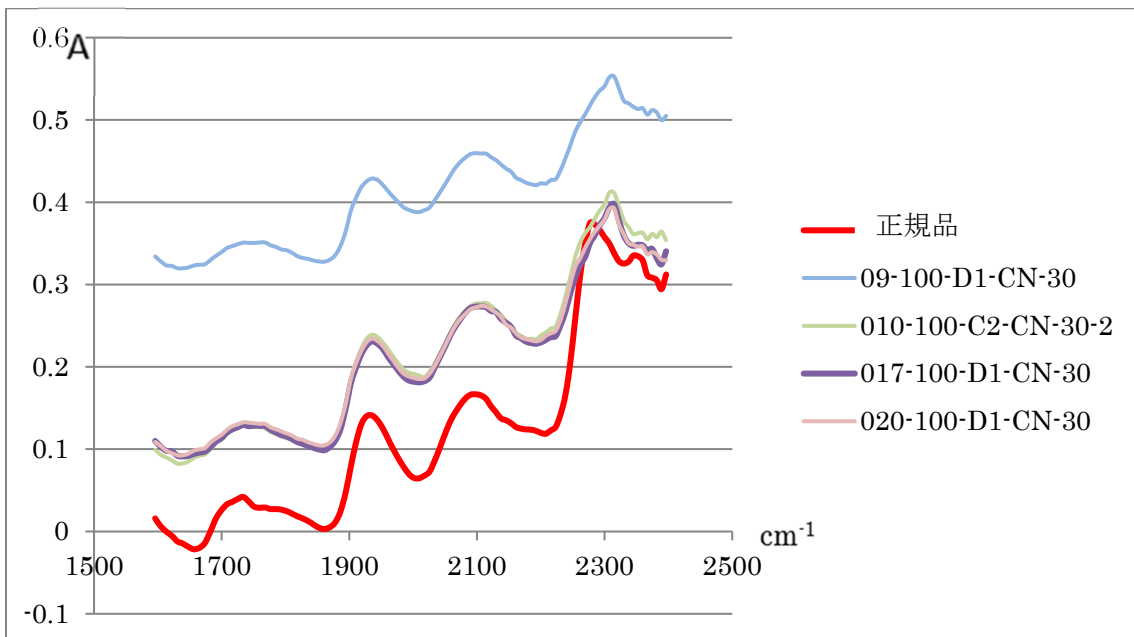
図 6-2 NIR の結果 (2) 100mg 模造品と 20mg 正規品の比較
