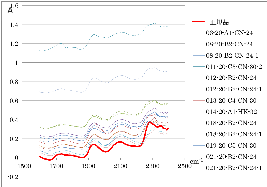
図 6-3 NIR の結果 (3) 20mg 模造品と 20mg 正規品の比較
