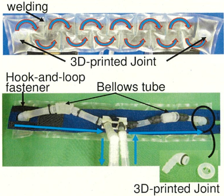
車椅子に搭載可能な冷却水循環装置
