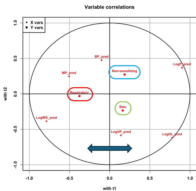
図3. 巨視的特徴量を用いた呼吸器・皮膚感作性に関するPLS-DA解析のローディングプロット
