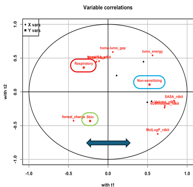
図2. 微視的特徴量を用いた呼吸器・皮膚感作性に関するPLS-DA解析のローディングプロット
