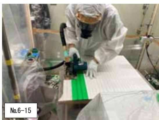
図 31-3 試験実施状況（スレート板）
