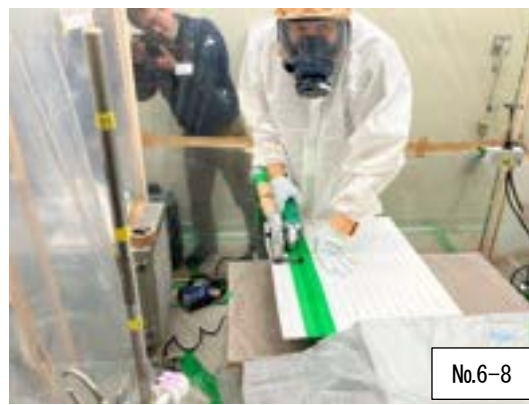
図 30-2 試験実施状況（スレート板）
