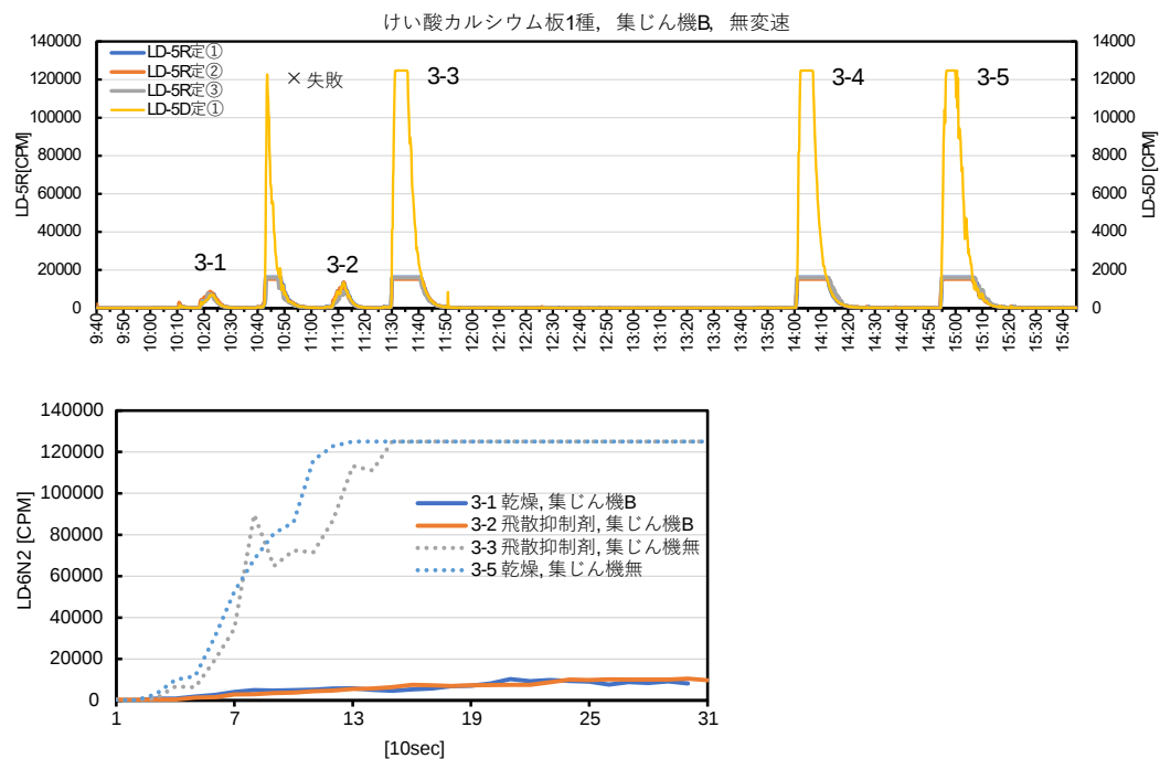
図 19-2 実験 3-1～3-5 の気中粒子相対濃度 (上図) 定点測定の時系列変化、(下図) 個人ばく露測定結果の比較 (No. 3-4 (水, 集じん機無) は、LD-6N2 エラーによりデータなし)
