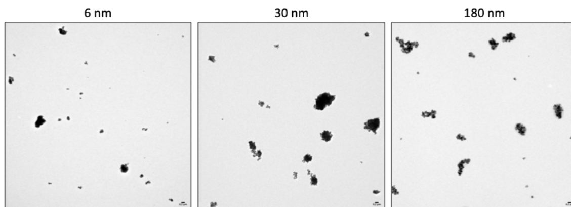
Figure 3. 本研究で用いた異なる結晶子径を持つ TiO 2 粒子の代表的透過電子顕微鏡像。
