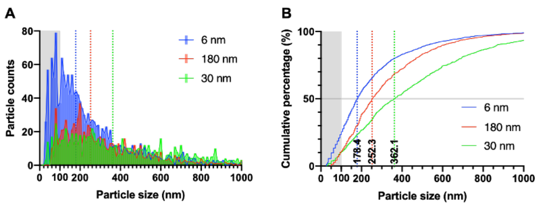
Figure 4. 異なる結晶子径を持つ TiO 2 粒子の透過電子顕微鏡観察による粒度分布(A)および積算粒度分布(B)。破線はメジアン径を示す。ナノ粒子 (> 100 nm) の分布を灰色で示した。
