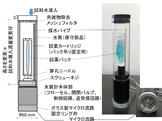
図9 簡素化水質計の構成と外観
