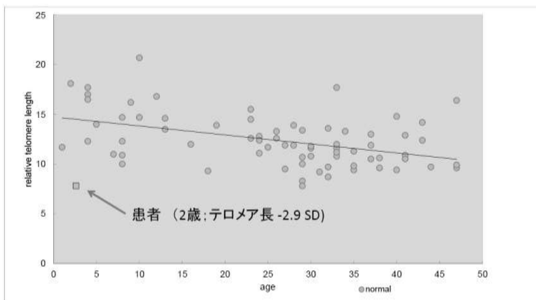
図 2. Flow-FISH 法によるテロメア長の測定
