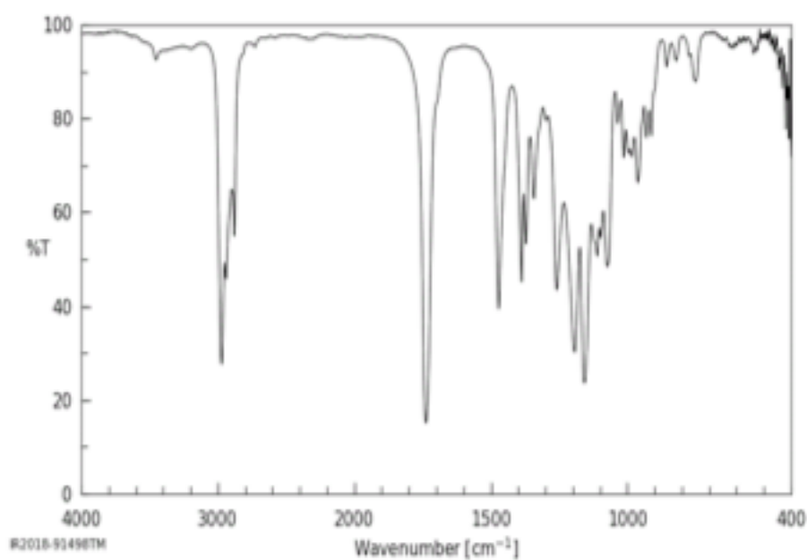
2,2,4-トリメチル-1,3-ペンタンジオールジイソブチレートの赤外吸収スペクトル 有機化合物のスペクトルデータベース SDBS 国立研究開発法人産業技術総合研究所 ( https://sdbb.db.aist.go.jp/sdbb/cgi-bin/direct_frame_top.cgi )
