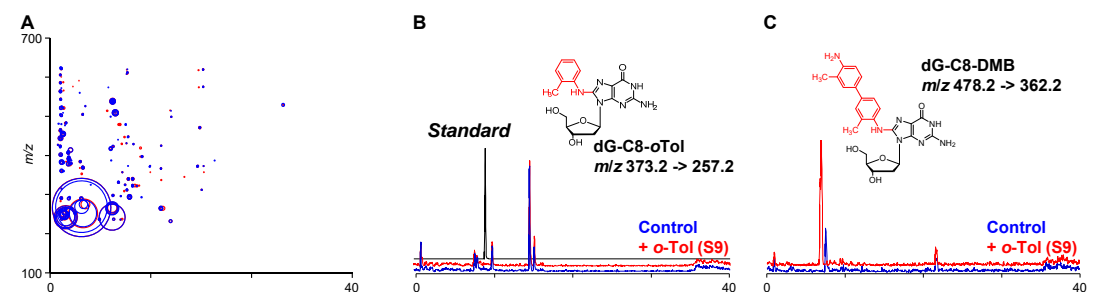
図2 o -Tol の S-9 mix 代謝物を曝露した calf thymus DNA のアダクトーム解析 (A) 検出された修飾ヌクレオシドのピーク面積をバブルの大きさで示したアダクトームマップ。横軸が保持時間縦軸が質量電荷比( m/z )。 (B) dG-C8- o Tol ( m/z 373.2>257.2) のMRMクロマトグラム。 (C) dG-C8-DMBの質量電荷比( m/z 478.2>362.2)に相当するMRMクロマトグラム。
