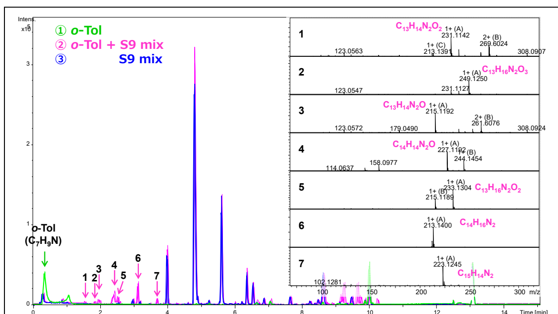
図1 o -Tol の S-9 mix 代謝物 LC-MS 分析で得られたクロマトグラム 右側は、ピーク1~7のMSスペクトルおよび組成式を示す。
