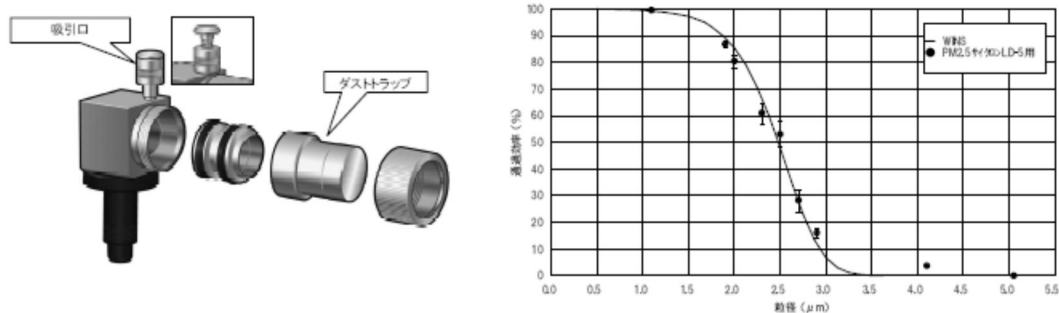
図3 - 4 PM2.5 サイクロンの構造 ( 左 ) と 1.7 L/min 吸引時の分離特性 ( 右 ) 元々の PM2.5 サイクロンは吸引口を閉塞できる構造となっていてインラインで使用できないので図2 - 5 のように入口部をストレートにした形態で別に作成した。
