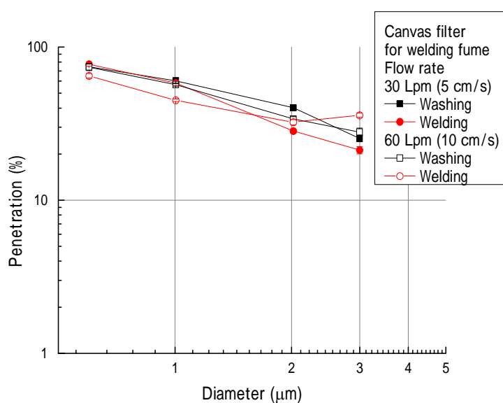
図 4 - 1 1 大型バグフィルタのろ布（織布）試料の通過率 使用後のろ布とそれを水洗した試料
