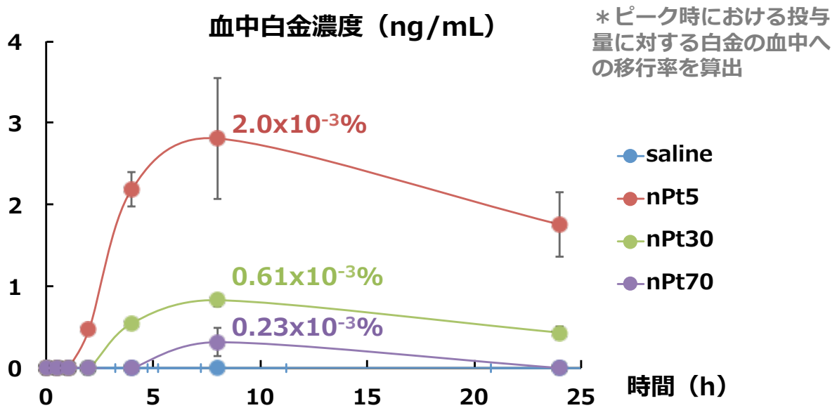
Figure 1 ナノ白金粒子の腸管吸収性. 雄性BALB/cマウス (8週齢) に、nPt5、nPt30、nPt70 (10 mg Pt/kg) を経口投与した。投与0、0.5、1、2、4、8、24時間後に血液を回収し、誘導結合プラズマ質量分析 (ICP-MS) により血中白金濃度を測定した。
