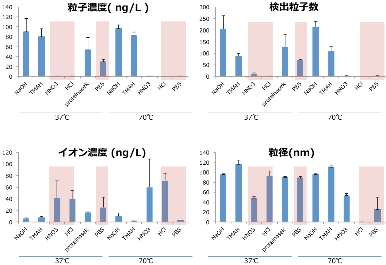
Figure 7 ICP-MSによるナノ銀粒子の臓器中での存在量・存在様式の解析. PBSにて10% (w/w) にホモジネートしたマウス肝臓に対して、銀粒子を200 ng/mLで添加した後、試料に水酸化ナトリウム、TMAH、硝酸、塩酸、proteinase Kの各溶液をそれぞれ1:1の割合で混和し、夾雑物の分解を試みた。この際、proteinase Kを除く3つの試薬については、37°Cと70°Cにて、proteinase Kについては37°Cにて、それぞれ3時間作用させた。各条件下のサンプルに対して、ICP-MSの時間分析モード（積分時間10 ms, 分析時間30 sec）にて、粒子径、粒子濃度、イオン濃度をそれぞれ測定した。
