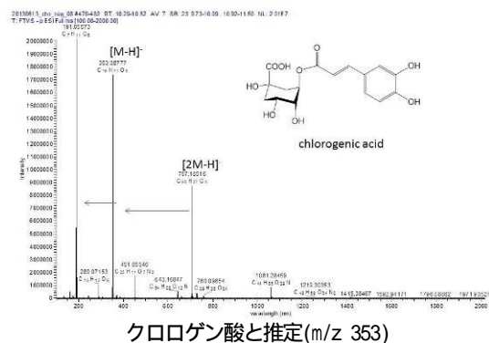
r. t. 10.0min 付近の TIC (左) と MS (右)
