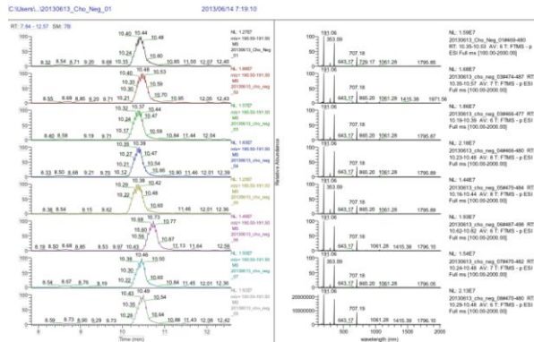
r. t. 10.0min 付近の TIC (左) と MS (右)
