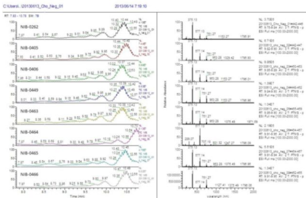
第1候補化合物 r. t. 9.66min 付近の TIC (左) と相当する MS (右) (negative mode)
