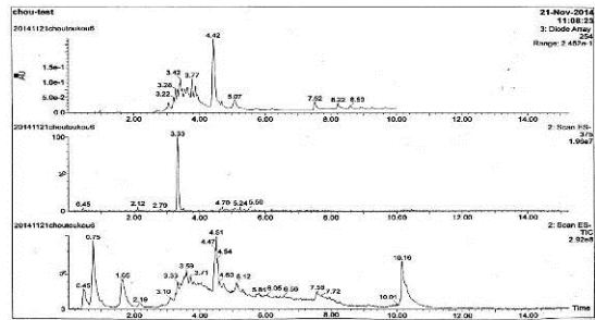
精製前熱水抽出エキスの LC/MS
