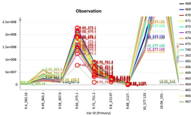
赤丸に該当する r. t. -m/z
