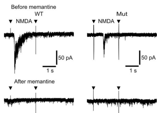
図3 野生型及び Grid2 変異マウスの小脳顆粒細胞の NMDAR 活性とメマンチンの影響
