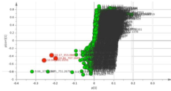
第2候補化合物の推定
