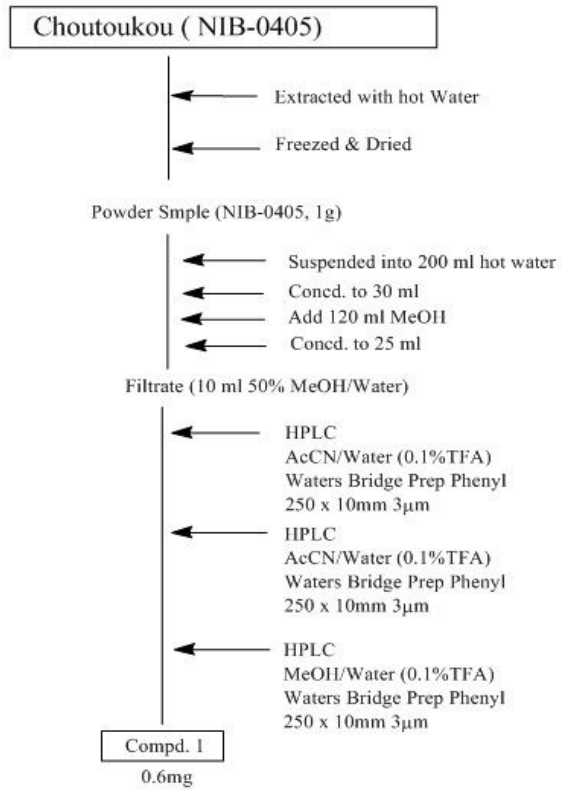
第 1 候補化合物 m/z375 の精製単離
