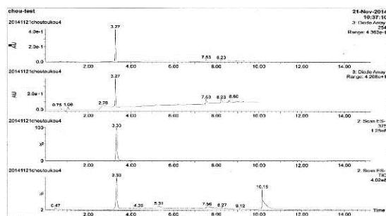
精製後の化合物の LCMS (waters 分取 LCMS)
