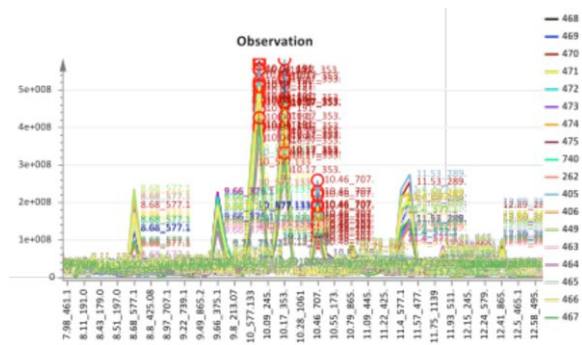
第2候補化合物の推定: r. t. 10.04_m/z191m, r. t. 10.17_m/z353, r. t. 10.46_m/z707
