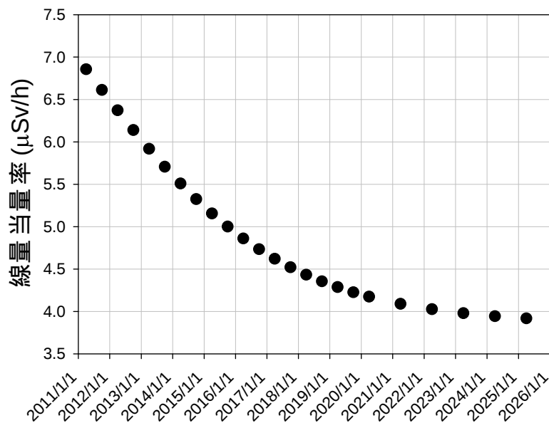
図 I.6 放射性セシウム濃度 500 Bq/g（地表面）を有する直径 30 cm の円形汚染土壌（計算モデル，緩衝深度：1.2 g/cm²（最小の線量当量率を与える））の中央高さ 5 cm における線量当量率の経時変化
