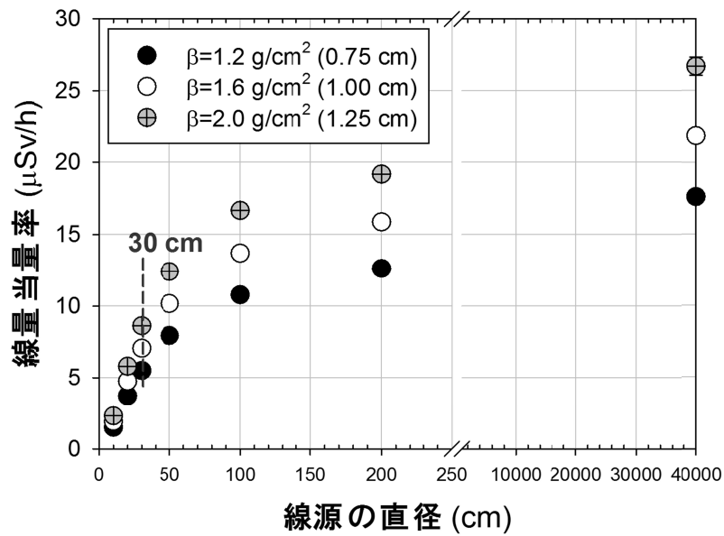
図 I.5 指数関数的な土壌中深さ分布を有する放射性セシウムの円形汚染土壌（計算モデル，地表面の放射能濃度：500 Bq/g（平成 26 年 4 月））の中央高さ 5 cm における線量当量率
