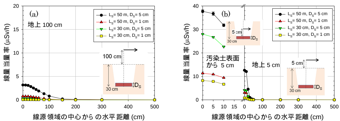
図 I.4 計算モデル（水路の堆積土）, 地上 100 cm 及び 5 cm における線量当量率 地表面の放射能濃度：500 Bq/g（平成 26 年 4 月）
