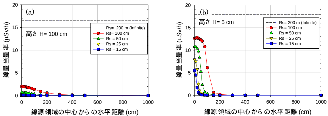
図 I.2 計算モデル（円形汚染）, 地上 100 cm 及び 5 cm における線量当量率 地表面の放射能濃度：500 Bq/g（平成 26 年 4 月）
