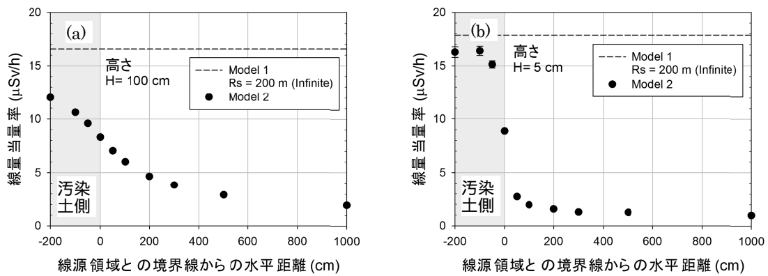
図 I.3 計算モデル（汚染土境界）, 地上 100 cm 及び 5 cm における線量当量率 地表面の放射能濃度：500 Bq/g（平成 26 年 4 月）
