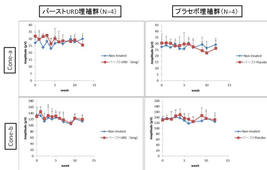
図 5 - 1 . Cone-ERG
