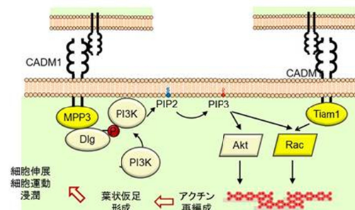
図 1 . CADM1 と PI3K を含む分子経路
