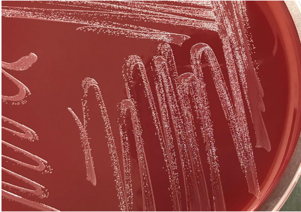
図 2-1 C. jejuni の集落
