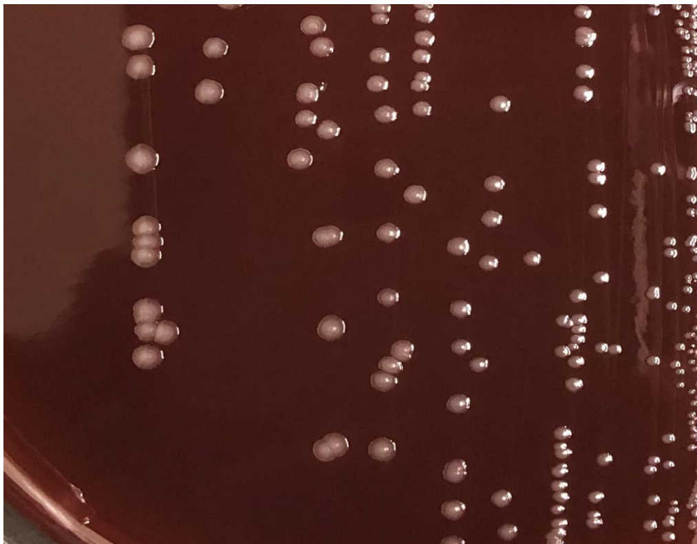
図 2-2 C. jejuni の集落
