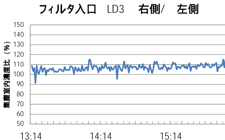
図4 - 5 帆布フィルタ上流左右の粉じん計の粉じん濃度比 粉じん入口と反対の右側の濃度が少し高い。
