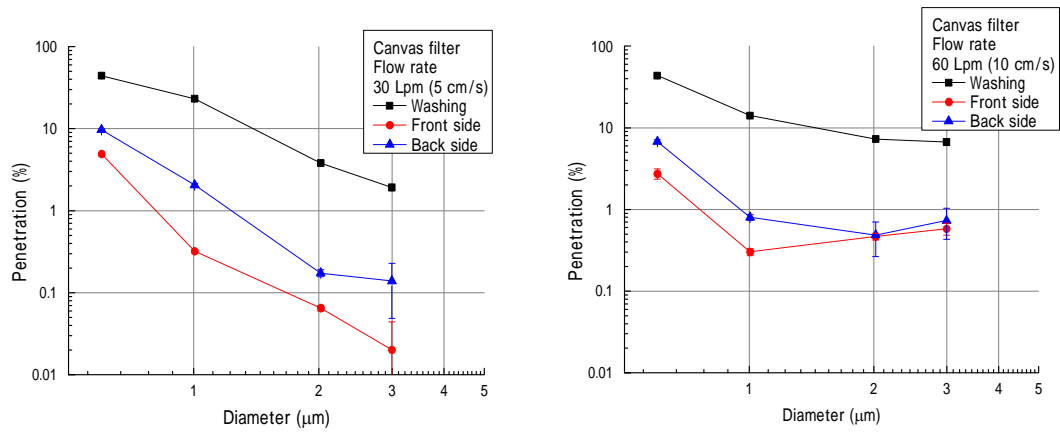
図 4 - 9 帆布フィルタの通過率 通過速度 5cm/s (左) と 10 cm/s (右)
