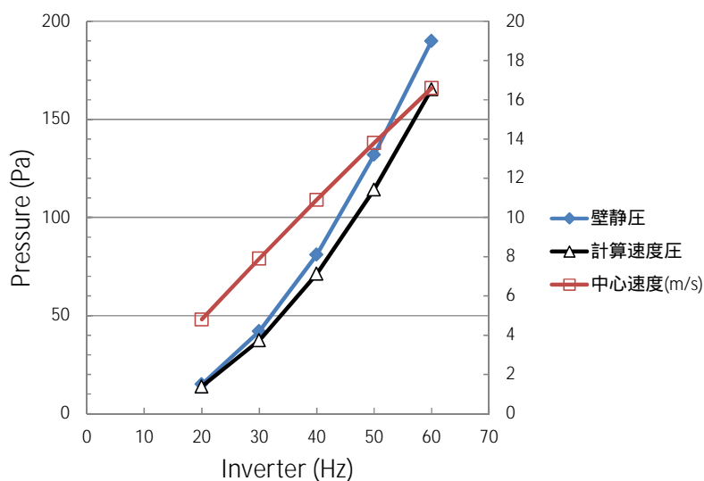
図 3 - 1 2 インバータ周波数とベルマウス下流静圧と熱線風速計によるダクト中心風速およびそれから計算される速度圧
