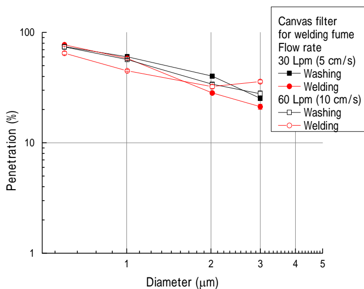
図 4 - 1 1 大型バグフィルタのろ布（織布）試料の通過率 使用後のろ布とそれを水洗した試料
