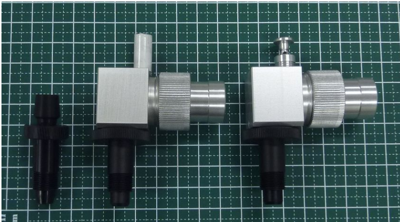
図3 - 2 本体から外したLD - 5 入口（左）とPM2.5 サイクロン（右） 中央はインライン吸入口
