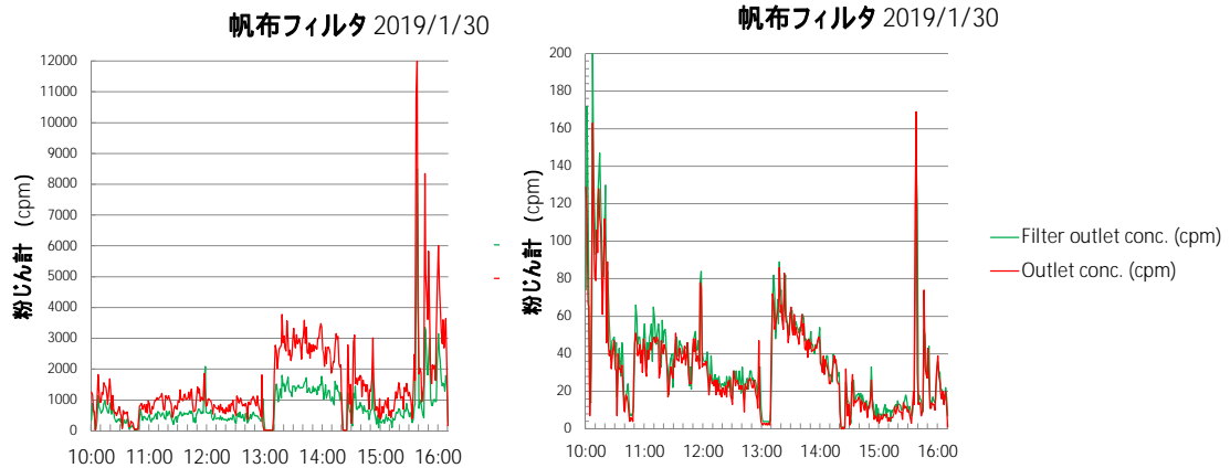
図 4 - 2 - 除じん装置前後と帆布フィルタ前後の粉じん計の粉じん濃度 (cpm 単位) 上流側濃度 (左) 下流側濃度 (右) 午後に石灰粉をフィーダーのホッパーに再供給するため 10 分間ほどの中断有
