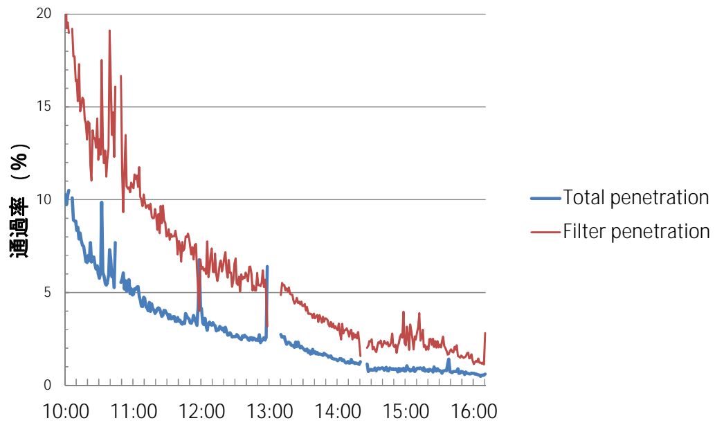
図4 - 1 除じん装置前後と帆布フィルタ前後の粉じん通過率の経時変化 1月30日新品から開始しての経過時間(単位は時分)
