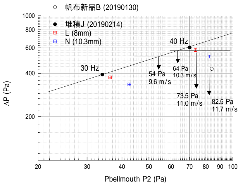
図 4 - 8 フィルタ取り付け部の漏れと入口速度圧（吸引風量の二乗）と圧力損失の関係 同じ圧力損失で吸引する場合の漏れの有無の推定方法として除じん装置のフィルタ部を通 過する風量（左）と漏れを含んだ全吸引風量（右）の組 流量から推定される漏れ率は隙間 8 mm で 6 %、隙間 10.3 mm で 18 %
