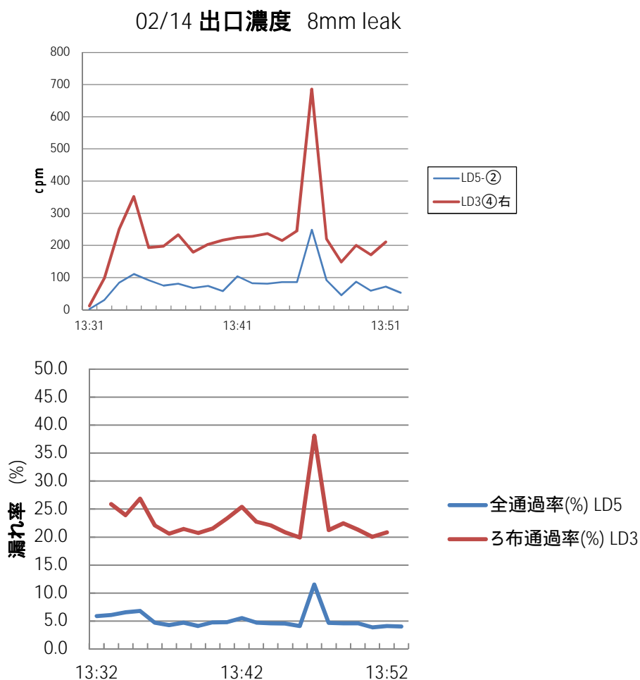
図4-6 隙間8mmでの除じん装置出口とろ布出口の濃度と漏れ率
