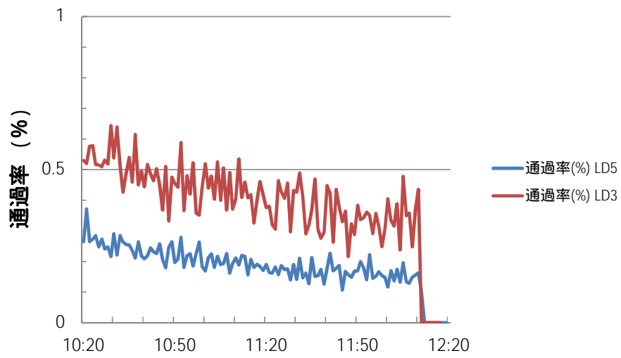
図4 -7 除じん装置入口と出口での通過率(LD-5)とろ布入口と出口での通過率(LD-3K)
