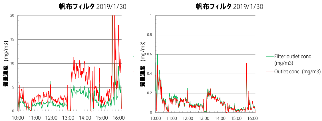
図 4 - 2 - 除じん装置前後と帆布フィルタ前後の粉じん計の粉じん濃度 (mg/m 3 単位) 上流側濃度 (左) 下流側濃度 (右) 午後に石灰粉をフィーダーホッパーに再供給するため 10 分間ほどの中断有 PM2.5 サイクロン付 LD-5 の質量濃度換算係数 (K 値) を 0.003 (mg/m 3 /cpm) とした。
