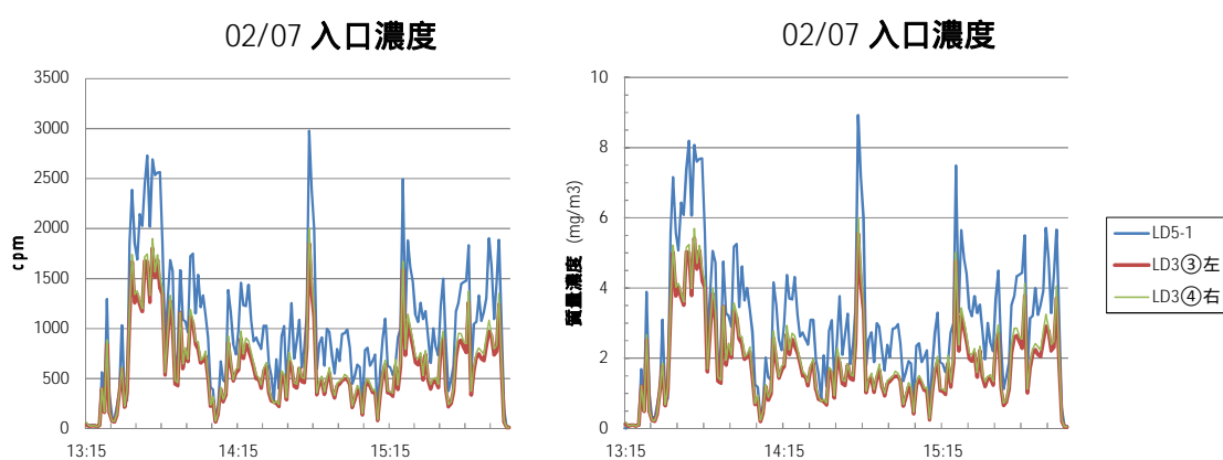
図4 - 4 除じん装置入口と帆布フィルタ上流左右の粉じん計の粉じん濃度 (cpm 単位、左) と (換算した質量濃度、右)
