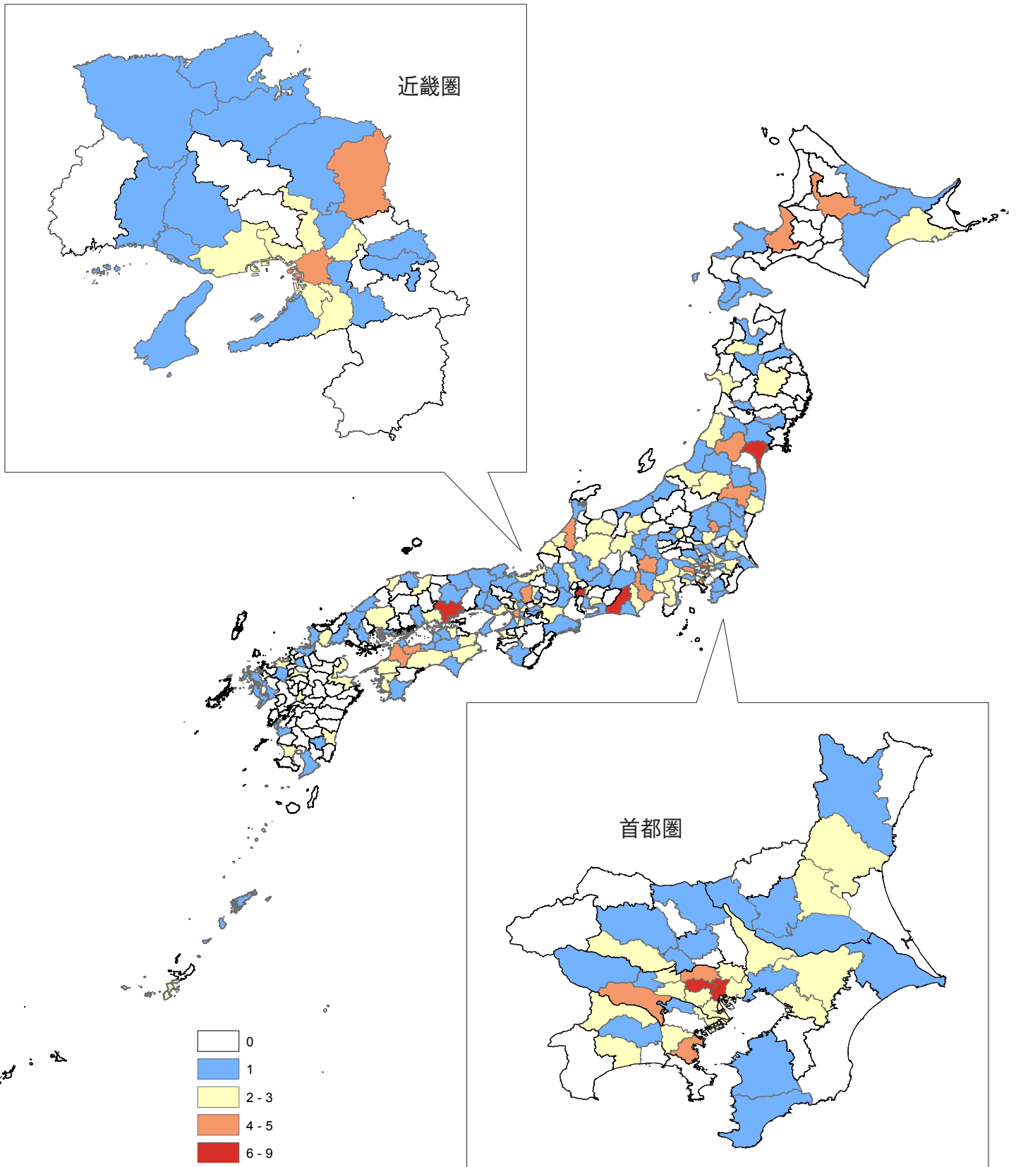
図2-2 全国の二次医療圏別の拠点病院数
