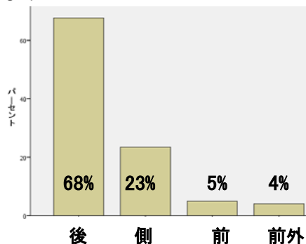
図3. 手術進入法(進入方向で分類)
