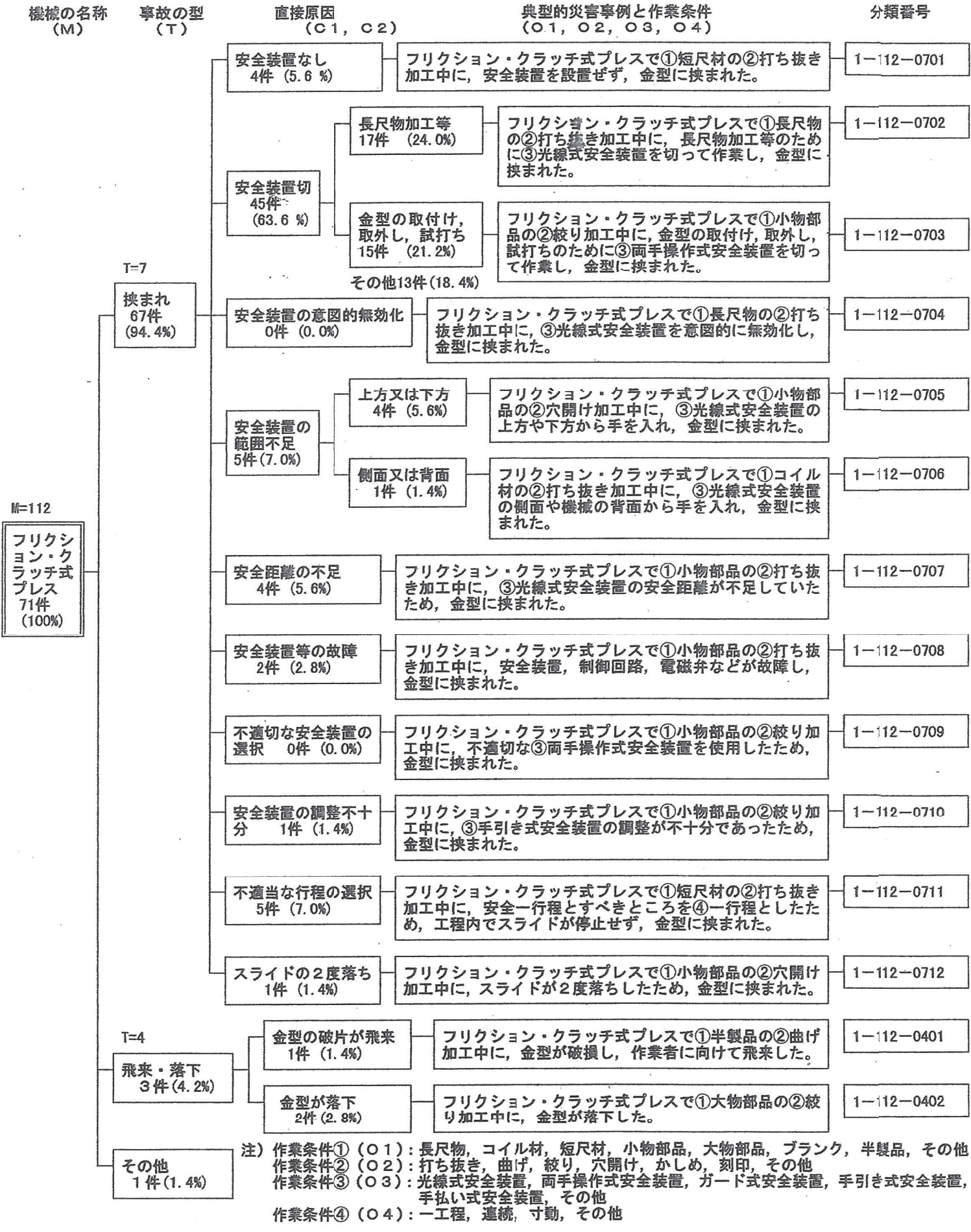
図 フリクシオン・クラッチ式プレスの典型的災害事例
