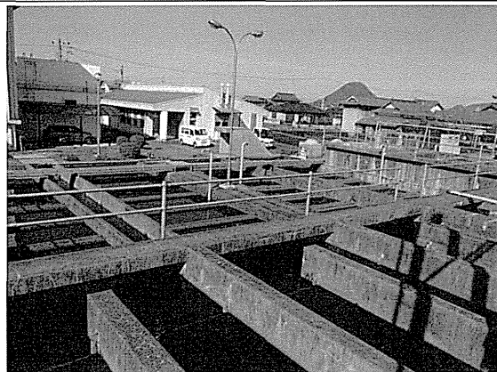
高速凝集沈澱池
