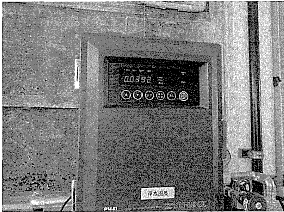
浄水濁度 (透過散乱光方式)
