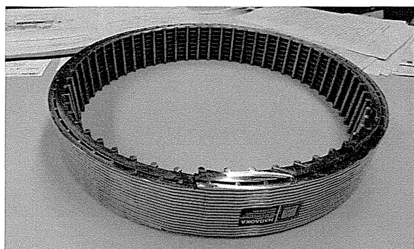
集水用スクリーン管のサンプル
