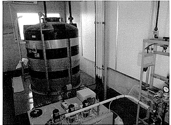
薬品タンク大 (次亜塩素)
