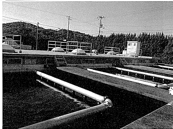
急速ろ過池 (地下は浄水池)
