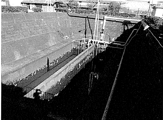
排泥池
