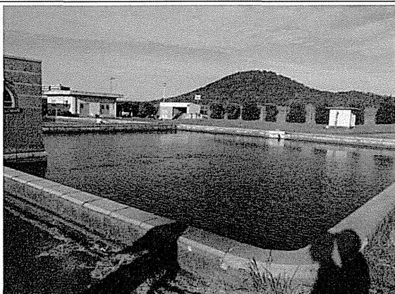
緩速ろ過池
