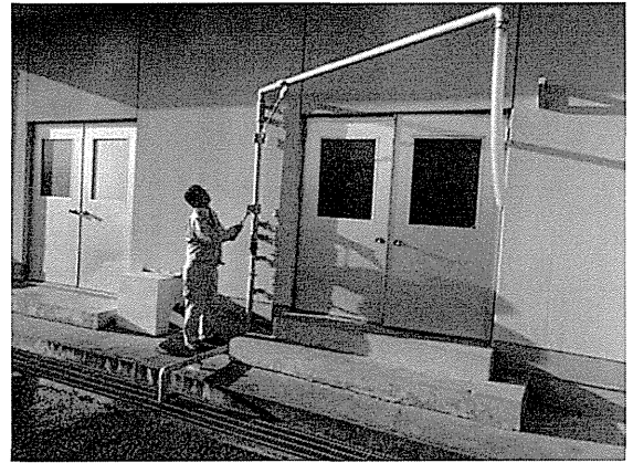
給水車注水用 (一人でもできる)
