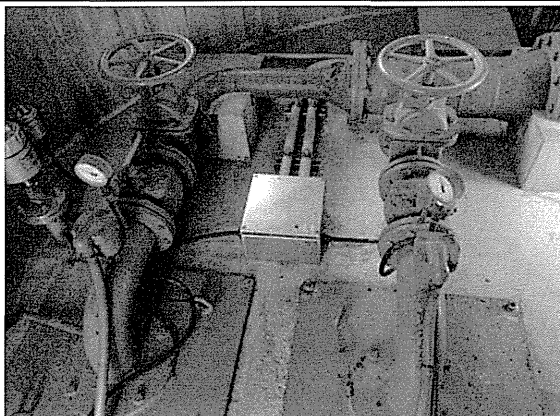
集水井内部
