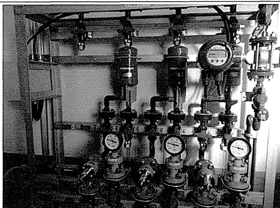
次亜塩素注入装置
