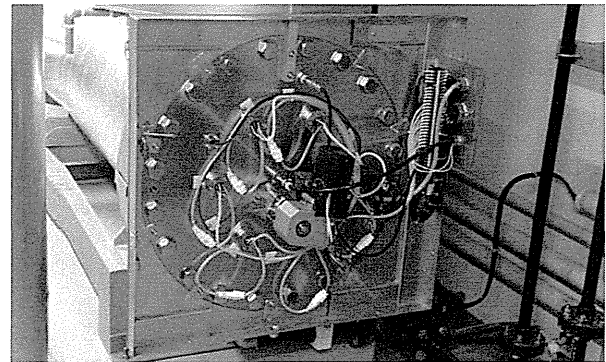
紫外線照射槽（端部カバーを外した状態）
