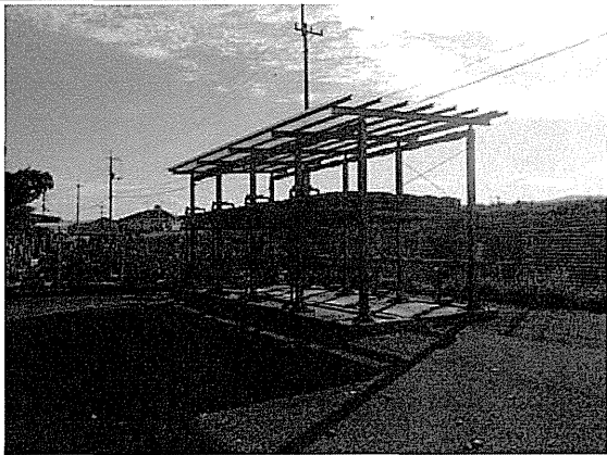
天日乾燥床
