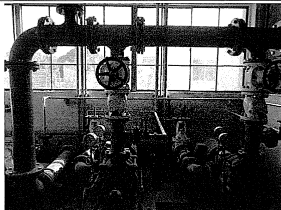
深井戸逆洗ポンプ
