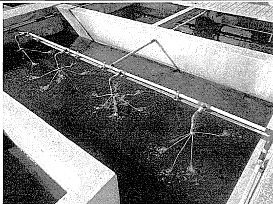
高速凝集沈澱池 (スラム防止)
