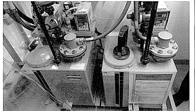
次亜注入ポンプ・小出し槽
