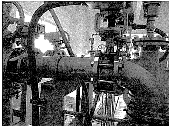
紫外線照射装置 (原水)
