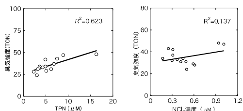
図8 水道水の臭気強度（カルキ臭を含む）と(左)TPN および(右)トリクロラミン濃度の比較
