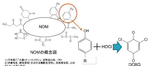
図 7 NOM からの HBQs の生成経路 (推測)
