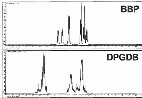
図9 BBPおよびDPGDBの NMR スペクトル ( \delta 6.5~8.5 ppm, メタノール- d_4 )
