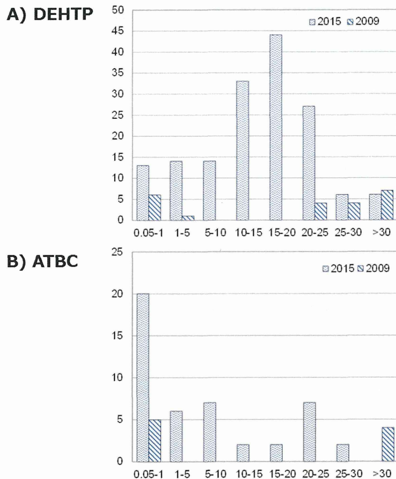
図3 2015および2009年度における各可塑剤の含有量の分布(指定外おもちゃ) A) DEHTP、B) ATBC、横軸:含有量(%), 縦軸:検体数
