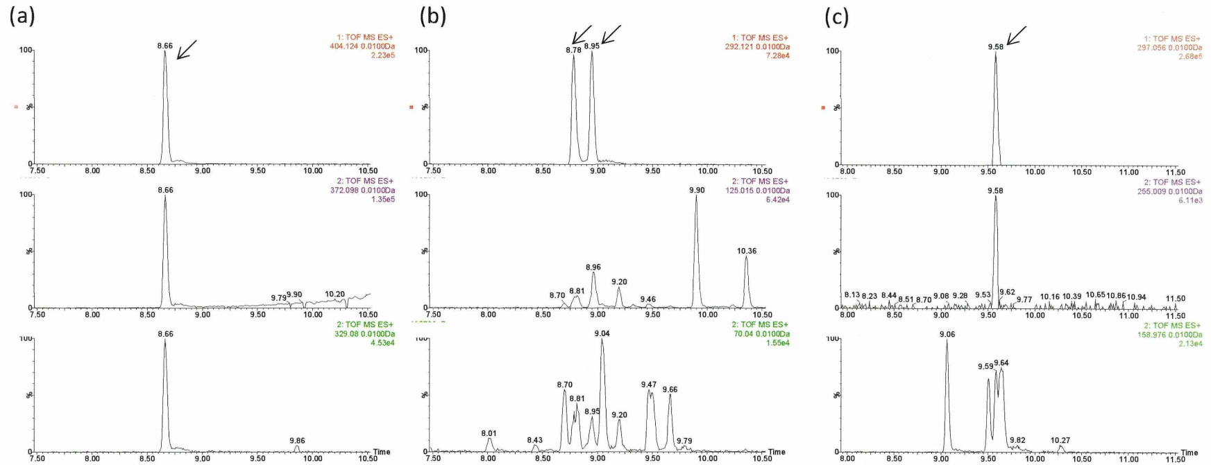
図5 標準溶液(0.01 \mu\text{g/mL} )における定量イオン及びそのフラグメントイオンの抽出イオンクロマトグラム(質量抽出幅 10 mDa)
