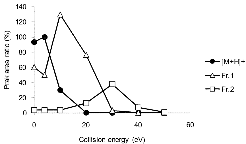
図 4 アゾキシストロビンとそのフラグメントイオン Fr.1 ( m/z 372.0979) 及び Fr.2 ( m/z 329.0795) のピーク面積に対するコリジョンエネルギーの影響 アゾキシストロビンのピーク面積の最大値を 100%と示した。 (キャピラリー電圧 1000 V、コロン電圧 20 V)
