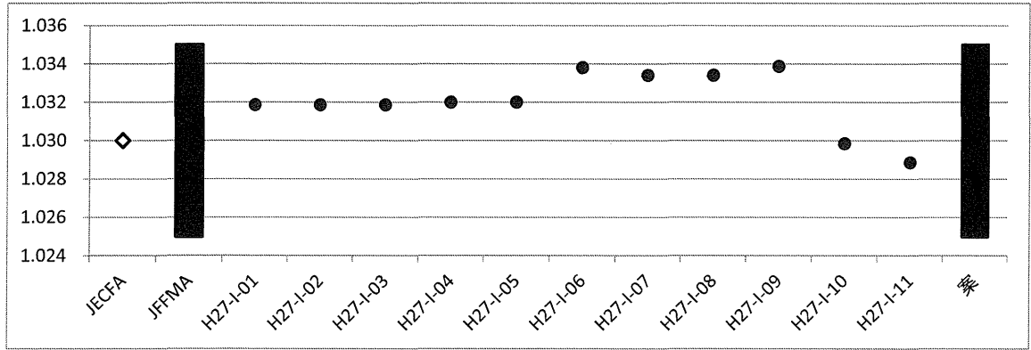
■□:規格(幅あり)、◆◇:規格(1点)、●○:実測値,それぞれ黒塗りは20℃、白抜きは25℃
