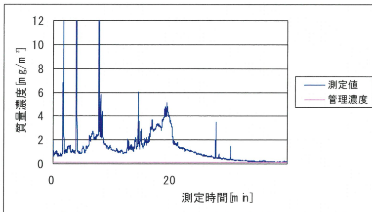
図 2.36 作業場 C における手込め作業 2 回目の粉じんばく露濃度変動
