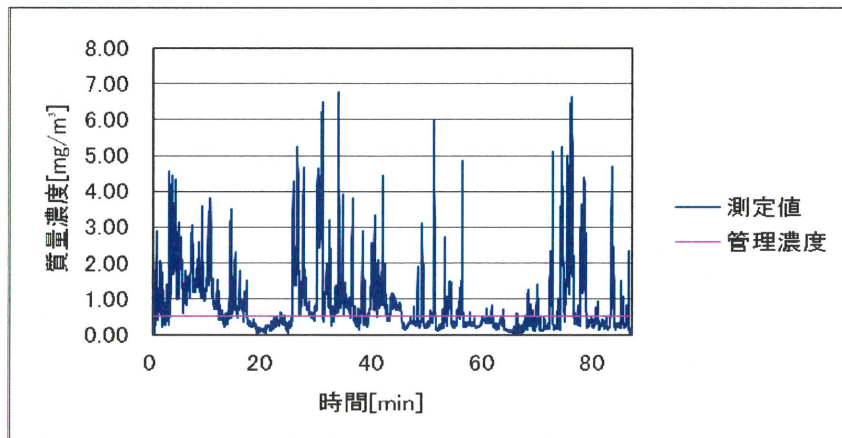
図 2.42 作業場 E における手込め作業 1 回目の粉じんばく露濃度変動
