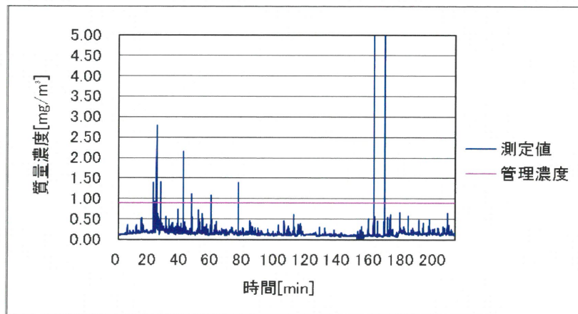
図 2.49 作業場 F における手込め作業 1 回目の粉じんばく露濃度変動
