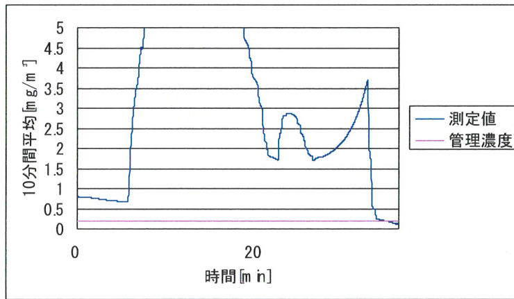
図 2.29 作業場 B における手込め作業 4 回目の粉じんばく露濃度変動 (10 分間移動平均値)
