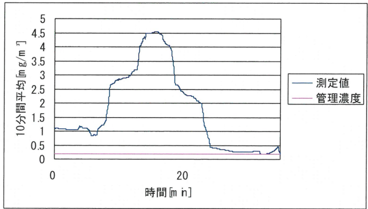
図 2.31 作業場 B における手込め作業 5 回目の粉じんばく露濃度変動 (10 分間移動平均値)
