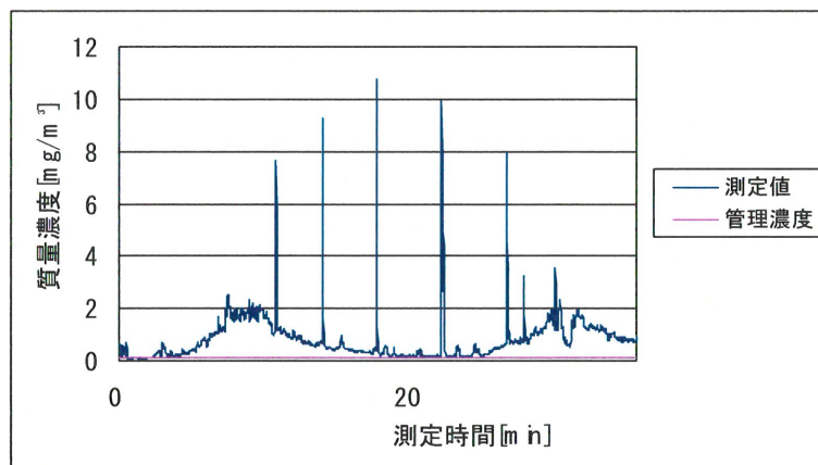
図 2.34 作業場 C における手込め作業 1 回目の粉じんばく露濃度変動
