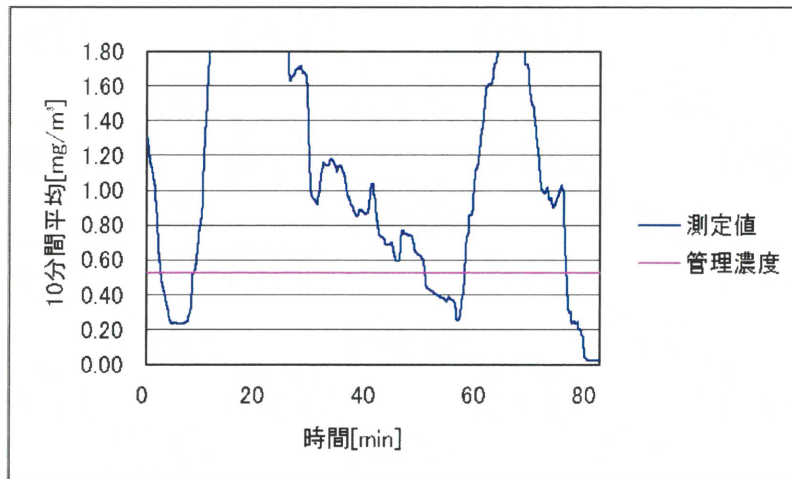
図 2.45 作業場 E における手込め作業 2 回目の粉じんばく露濃度変動 (10 分間移動平均値)
