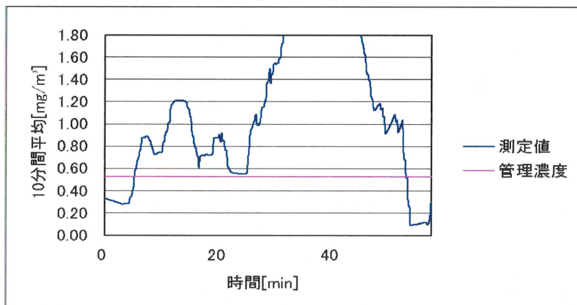
図 2.47 作業場 E における手込み作業 3 回目の粉じんばく露濃度変動 (10 分間移動平均値)
