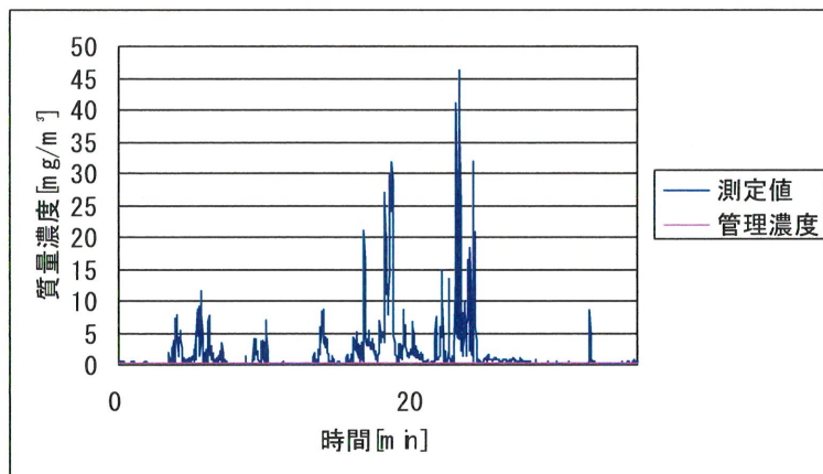
図 2.30 作業場 B における手込め作業 5 回目の粉じんばく露濃度変動
