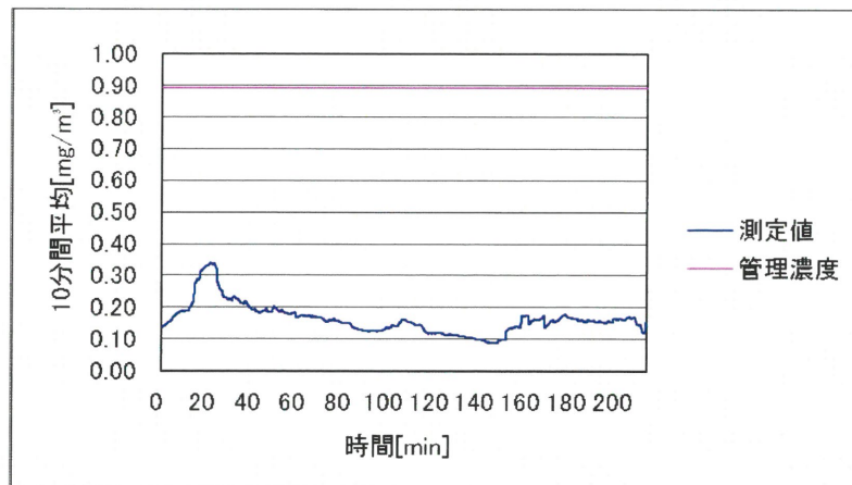
図 2.50 作業場 F における手込め作業 1 回目の粉じんばく露濃度変動 (10 分間移動平均値)
