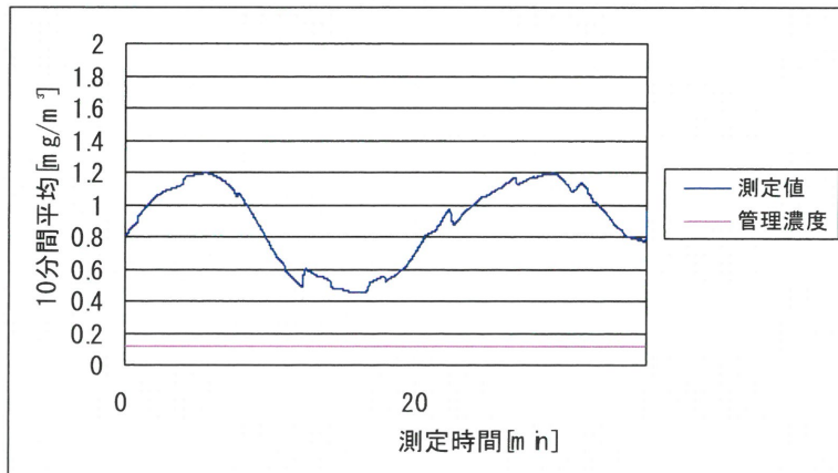
図 2.35 作業場 C における手込め作業 1 回目の粉じんばく露濃度変動 (10 分間移動平均値)
