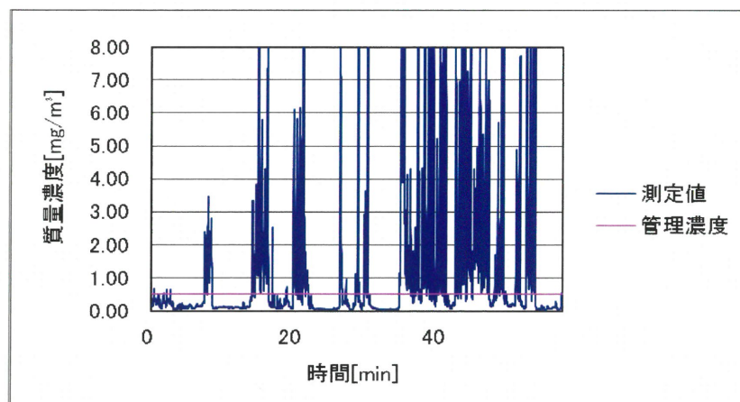
図 2.46 作業場 E における手込め作業 3 回目の粉じんばく露濃度変動
