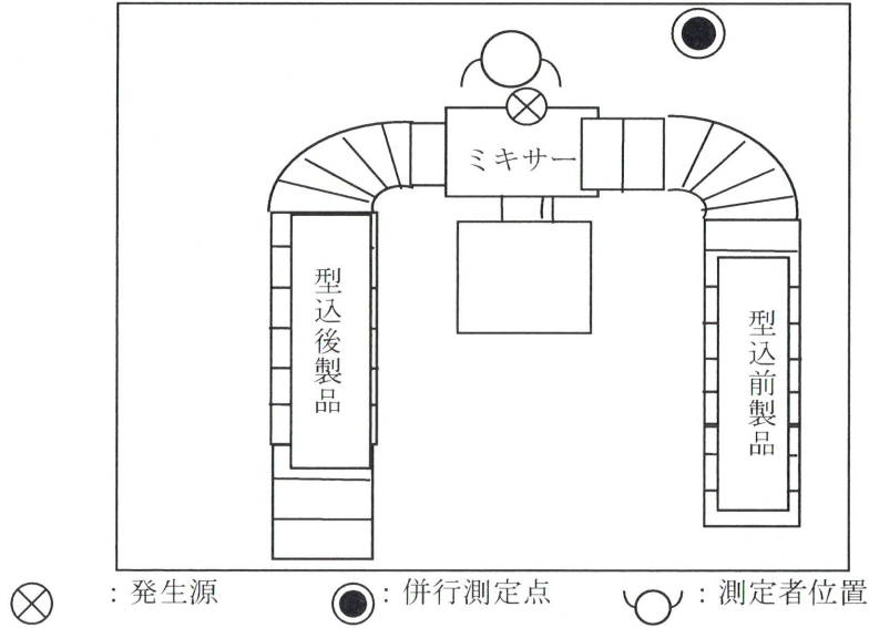
図 2.38 作業場Dの概略図
