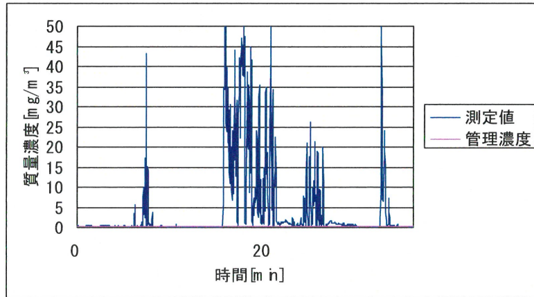
図 2.28 作業場 B における手込め作業 4 回目の粉じんばく露濃度変動
