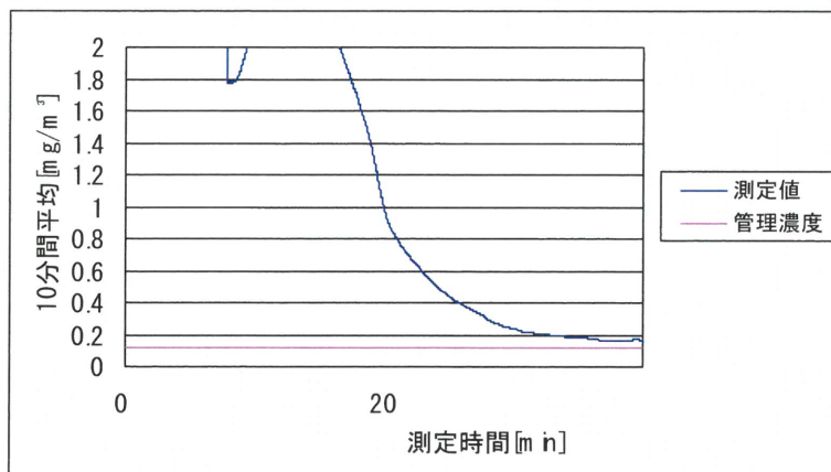
図 2.37 作業場 C における手込め作業 2 回目の粉じんばく露濃度変動 (10 分間移動平均値)
