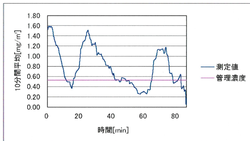
図 2.43 作業場 E における手込め作業 1 回目の粉じんばく露濃度変動 (10 分間移動平均値)
