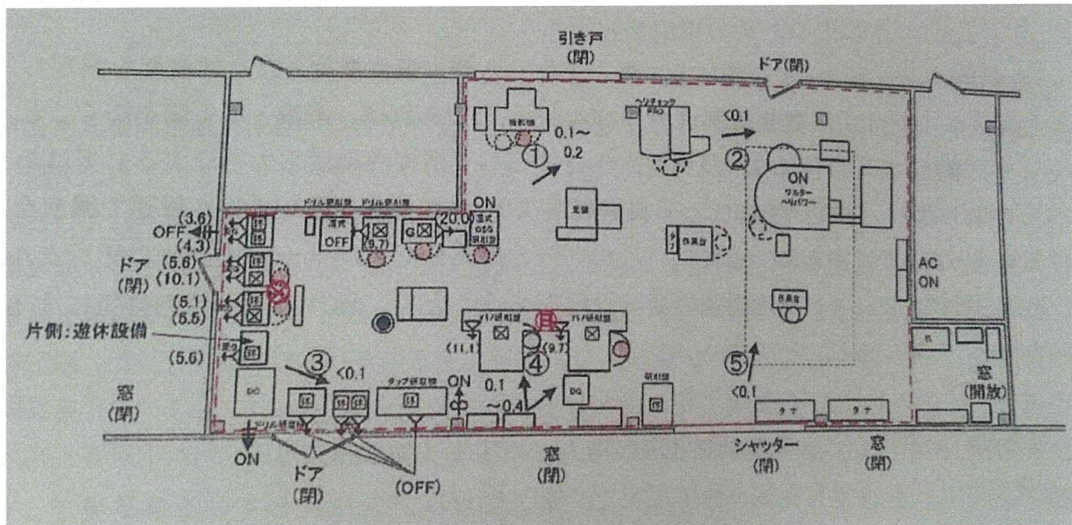
図 4.74 測定対象作業場の概略
