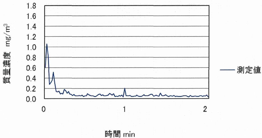
図 4.85 キャノピー式フードを通常の半分の吸引風速で稼働した時の粉じん漏洩濃度の時間的変動状況
