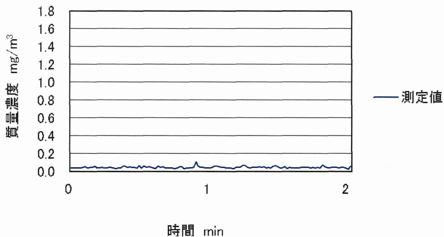
図 4.84 キャンピー式フードを通常の吸引風速で稼働した時の粉じん漏洩濃度の時間的変動状況
