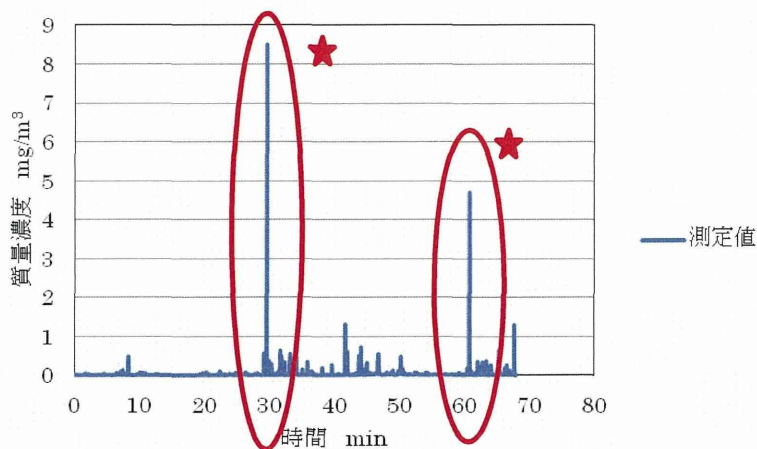
図 4.94 囲い式フードを通常時の 3 分の 2 の吸引風速で稼働した時の粉じんばく露濃度の変動状況
