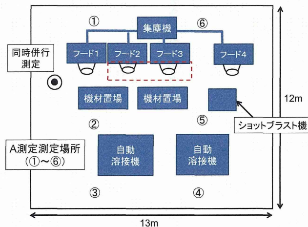
図 4.98 作業場の概略図
