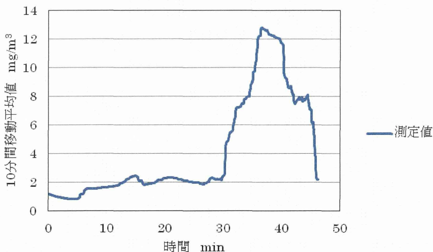
図 4.105 囲い式フードを通常時の吸引風速で稼働した時のフード3で従事していた作業者の粉じんばく露濃度 (10分間移動平均値)
