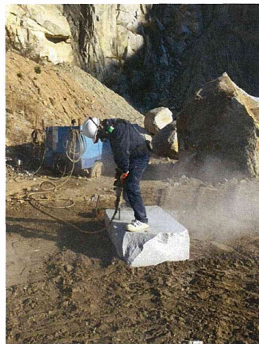
図 2.12 小割り作業状況 (その2)
