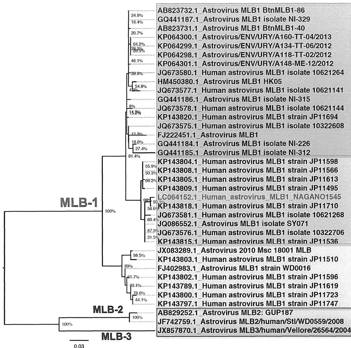
図12 Human astrovirus の分子系統解析。分子系統解析で分類に使用される RNA-dependent RNA polymerase 遺伝子の部分配列を抽出し (LC064152.1|Human_astrovirus_MLB1_NAGANO1545, 3173-3495: 323 nt)、1,000 回ブートストラップを加えた最尤法にて分子系統樹を作成し評価した。スケールバーは塩基当たり 0.03 箇所の置換を示す。ブランチにブートストラップ値を示す。
