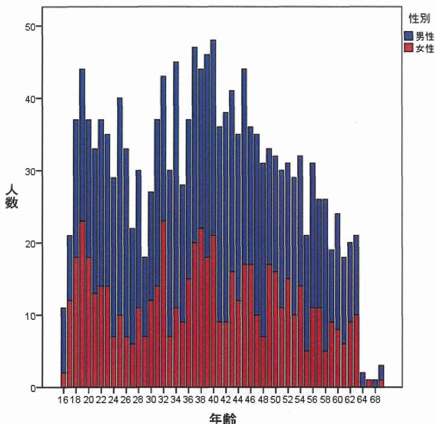
図2 問診該当①による不適格者の性・年齢階級別分布
