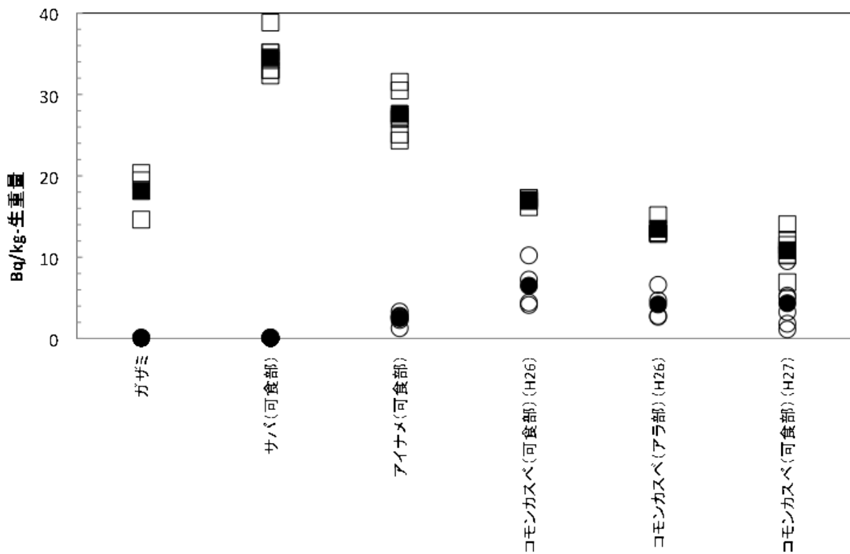
図 1 同一魚種の個体毎の ^{137}\text{Cs} 及び ^{40}\text{K} 濃度差について。
