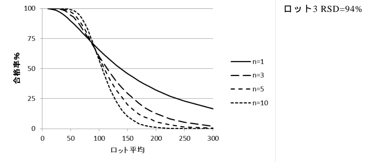
図5 シイタケロットからの計量基準型サンプリングのOC曲線
