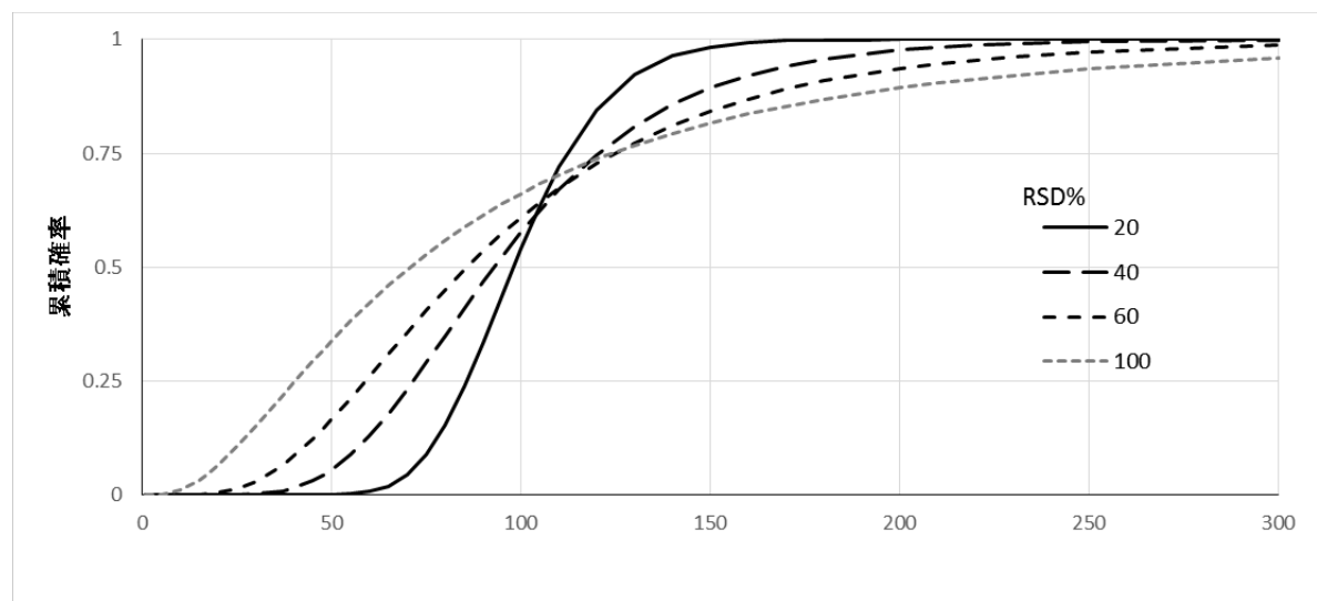
図2 対数正規分布の確率密度と累積確率 平均値は100とした。
