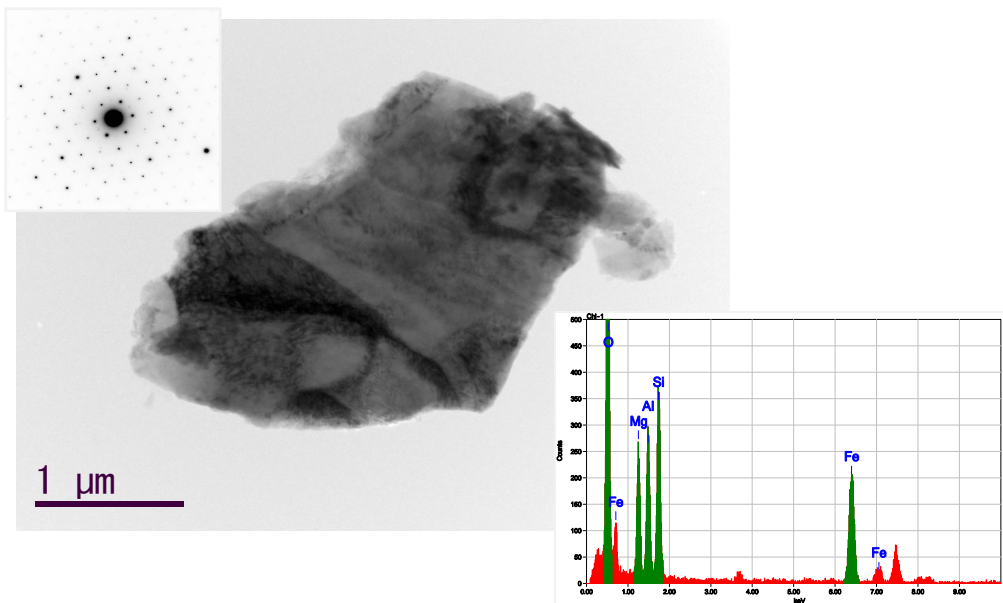
写真 10 . 緑泥石の TEM 写真 (左上 : 電子回折パターン、右下 : EDS スペクトル)
