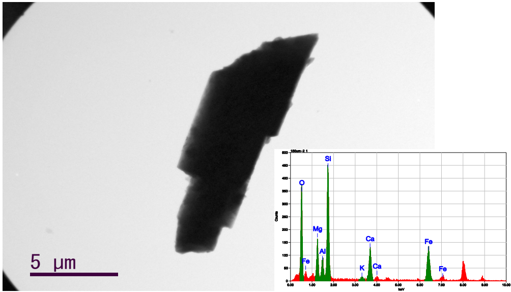
写真 9 . 角閃石の TEM 写真と EDS スペクトル
