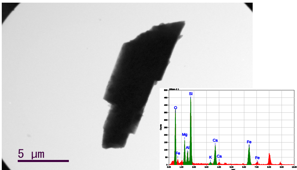
写真 1 . 角閃石の TEM 写真と EDS スペクトル
