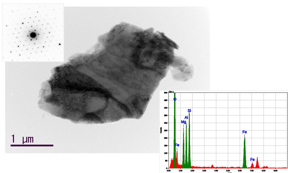
写真 2 . 緑泥石の TEM 写真 (左上：電子回折パターン、右下：EDS スペクトル)
