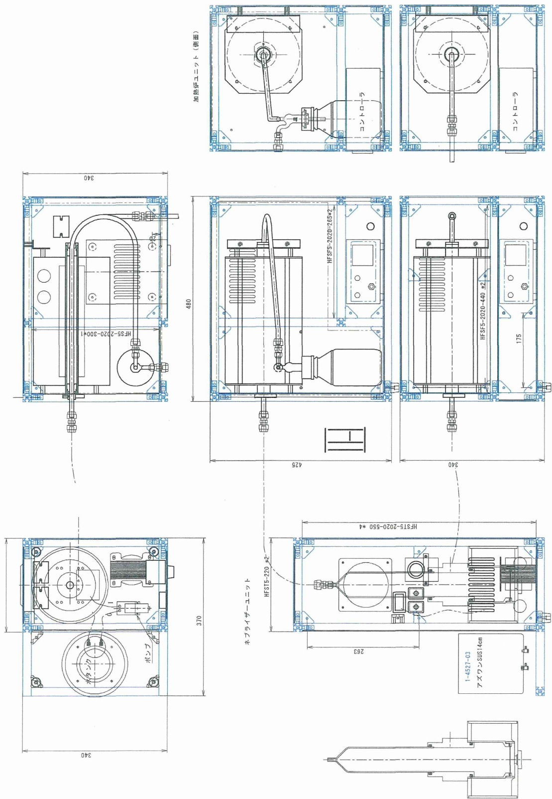
図 10 有機質・無機質繊維除去処理装置の概要 (図面)
