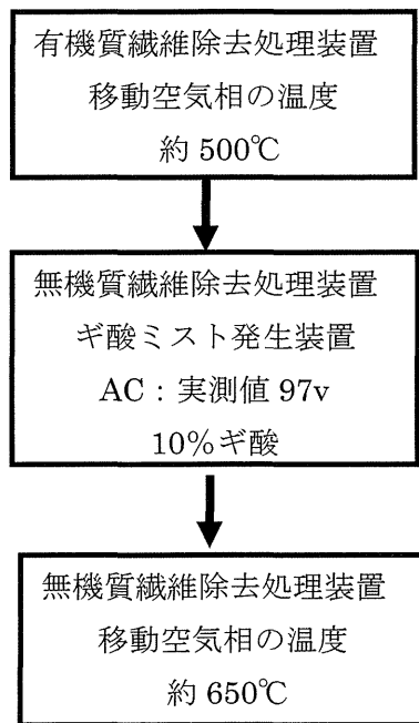
図 11 有機質・無機質繊維除去処理装置の構成
