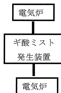
図 9 3ブロック方式による有機質・無機質除去処理装置の構成
