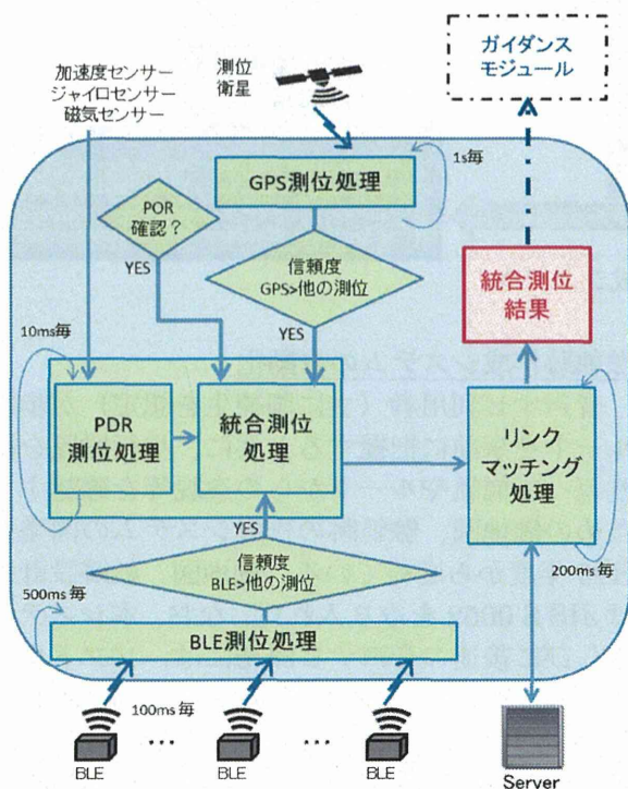
図 4：統合測位エンジンの概略
