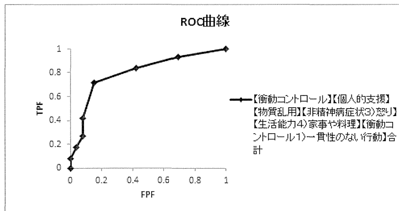
図 22 【衝動コントロール】【個人的支援】【物質乱用】【非精神病症状3) 怒り】【生活能力4) 家事や料理】【衝動コントロール1) 一貫性のない行動】の6項目合計による3年以内の問題行動予測のROC曲線
