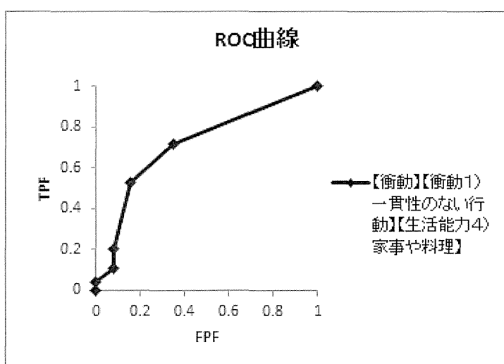
図 19 【衝動コントロール】【生活能力4) 家事や料理】【衝動コントロール1) 一貫性のない行動】合計得点による3年以内の問題行動予測のROC曲線
