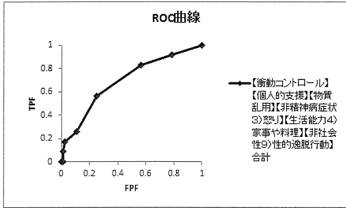
図 35 【衝動コントロール】 【個人的支援】 【物質乱用】 【非精神病症状 3) 怒り】 【生活能力 4) 家事や料理】 【非社会性 9) 性的逸脱行動】 の 6 項目合計による 2 年追跡した事例の問題行動予測の ROC 曲線
