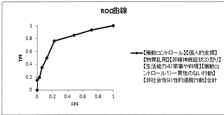
図 32 【衝動コントロール】【個人的支援】【物質乱用】【非精神病症状3) 怒り】【生活能力4) 家事や料理】【衝動コントロール1) 一貫性のない行動】【非社会性9) 性的逸脱行動】の7項目合計による3年以内の暴力予測のROC曲線
