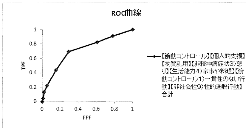
図 31 【衝動コントロール】【個人的支援】【物質乱用】【非精神病症状3）怒り】【生活能力4）家事や料理】【衝動コントロール1）一貫性のない行動】【非社会性9）性的逸脱行動】の7項目合計による2年追跡した事例の問題行動予測のROC曲線
