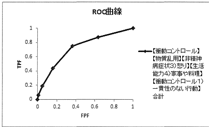
図 29 【衝動コントロール】【物質乱用】【非精神病症状3）怒り】【生活能力4）家事や料理】【衝動コントロール1）一貫性のない行動】の5項目合計による2年追跡した事例の暴力予測のROC曲線
