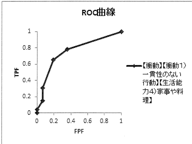
図 20 【衝動コントロール】 【生活能力 4) 家事や料理】 【衝動コントロール 1) 一貫性のない行動】 合計得点による 3 年以内の暴力予測の ROC 曲線
