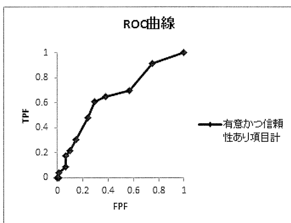
図 17 項目ごとのCOX比例ハザードモデルないし生存曲線の群間比較において通院移行後の問題行動の予測に効果が認められた項目から級内相関0.6未満の項目を除いた合計点による2年追跡した事例の問題行動予測のROC曲線
