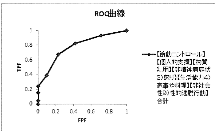
図 36 【衝動コントロール】 【個人的支援】 【物質乱用】 【非精神病症状 3) 怒り】 【生活能力 4) 家事や料理】 【非社会性 9) 性的逸脱行動】 の 6 項目合計による 3 年以内の暴力予測の ROC 曲線
