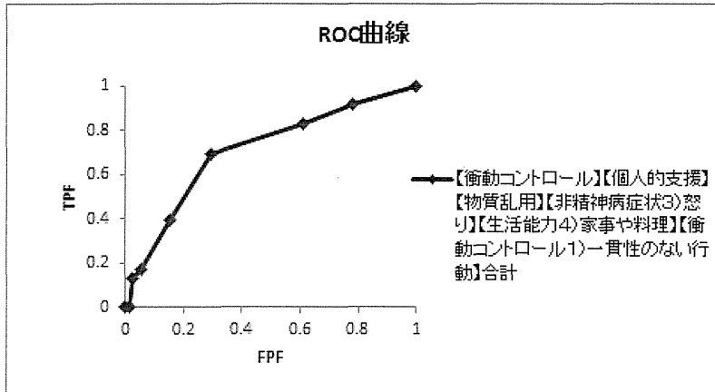
図 23 【衝動コントロール】【個人的支援】【物質乱用】【非精神病症状3) 怒り】【生活能力4) 家事や料理】【衝動コントロール1) 一貫性のない行動】の6項目合計による2年追跡した事例の問題行動予測のROC曲線
