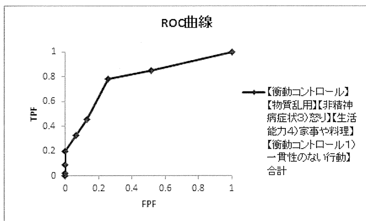
図 28 【衝動コントロール】【物質乱用】【非精神病症状3) 怒り】【生活能力4) 家事や料理】【衝動コントロール1) 一貫性のない行動】の5項目合計による3年以内の暴力予測のROC曲線
