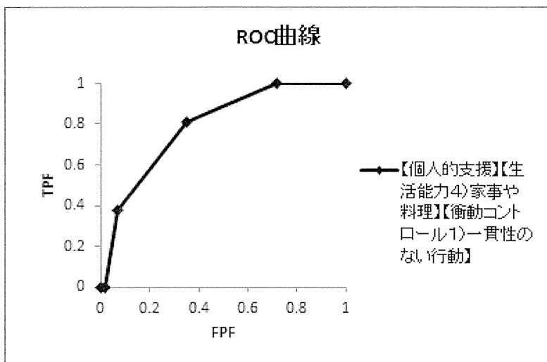
図 16 【個人的支援】【生活能力4)家事や料理】【衝動コントロール1)一貫性のない行動】合計得点による2年追跡した事例の暴力予測のROC曲線
