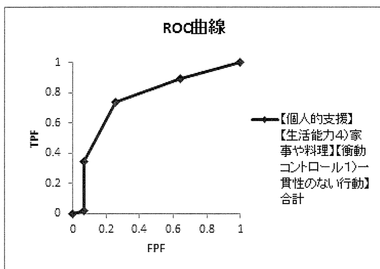
図 15 【個人的支援】【生活能力4) 家事や料理】【衝動コントロール1) 一貫性のない行動】 合計得点による3年以内の暴力予測のROC曲線
