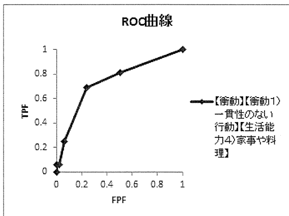
図 21 【衝動コントロール】 【生活能力 4) 家事や料理】 【衝動コントロール 1) 一貫性のない行動】 合計得点による 2 年追跡した事例の暴力予測の ROC 曲線
