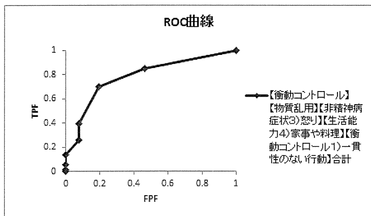
図 26 【衝動コントロール】 【物質乱用】 【非精神病症状 3) 怒り】 【生活能力 4) 家事や料理】 【衝動コントロール 1) 一貫性のない行動】 の 5 項目合計による 3 年以内の問題行動予測の ROC 曲線
