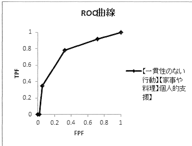
図 13 2年追跡した事例の問題行動予測のROC曲線
