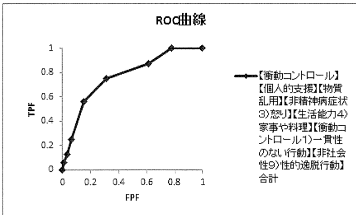
図 33 【衝動コントロール】【個人的支援】【物質乱用】【非精神病症状3) 怒り】【生活能力4) 家事や料理】【衝動コントロール1) 一貫性のない行動】【非社会性9) 性的逸脱行動】の7項目合計による2年追跡した事例の暴力予測のROC曲線
