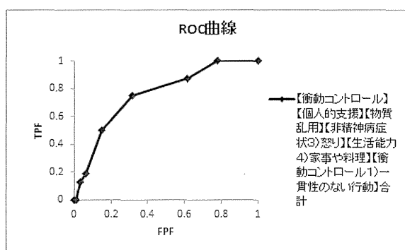
図 25 【衝動コントロール】【個人的支援】【物質乱用】【非精神病症状3) 怒り】【生活能力4) 家事や料理】【衝動コントロール1) 一貫性のない行動】の6項目合計による2年追跡した事例の暴力予測のROC曲線
