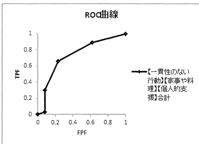
図 14 【個人的支援】【生活能力4) 家事や料理】【衝動コントロール1) 一貫性のない行動】 合計得点による3年以内の問題行動予測のROC曲線
