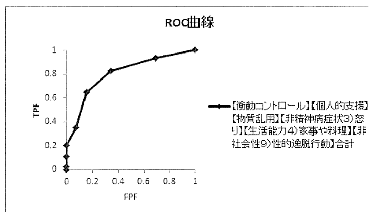
図 34 【衝動コントロール】【個人的支援】【物質乱用】【非精神病症状3) 怒り】【生活能力4) 家事や料理】【非社会性9) 性的逸脱行動】の6項目合計による3年以内の問題行動予測のROC曲線
