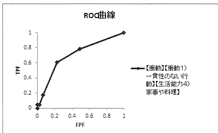
図 18 【衝動コントロール】【生活能力4)家事や料理】【衝動コントロール1)一貫性のない行動】合計得点による2年追跡した事例の問題行動予測のROC曲線
