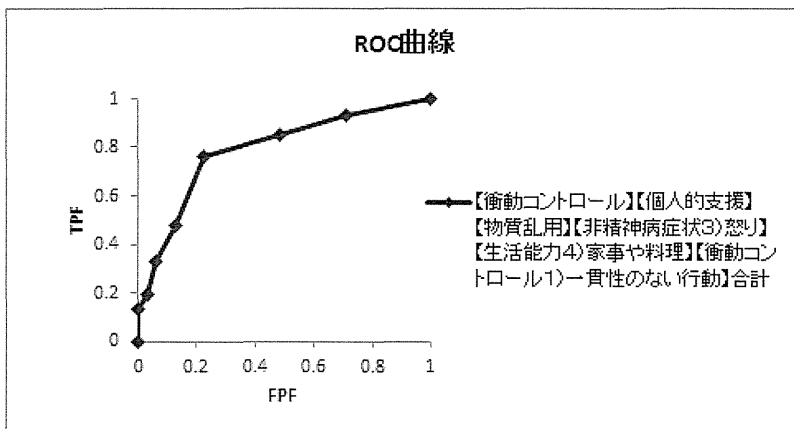
図 24 【衝動コントロール】【個人的支援】【物質乱用】【非精神病症状3) 怒り】【生活能力4) 家事や料理】【衝動コントロール1) 一貫性のない行動】の6項目合計による3年以内の暴力予測のROC曲線
