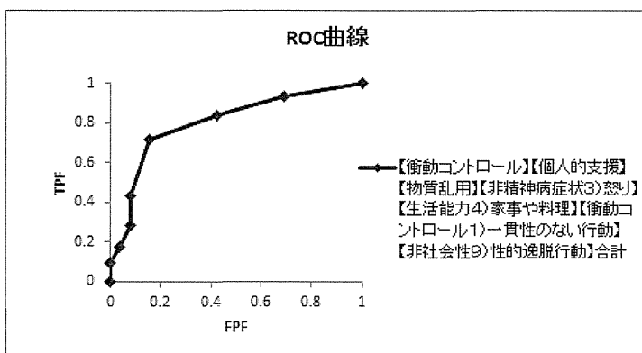
図 30 【衝動コントロール】【個人的支援】【物質乱用】【非精神病症状3）怒り】【生活能力4）家事や料理】【衝動コントロール1）一貫性のない行動】【非社会性9）性的逸脱行動】の7項目合計による3年以内の問題行動予測のROC曲線
