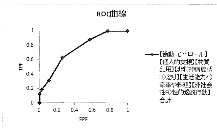
図 37 【衝動コントロール】【個人的支援】【物質乱用】【非精神病症状 3) 怒り】【生活能力 4) 家事や料理】【非社会性 9) 性的逸脱行動】の 6 項目合計による 2 年追跡した事例の暴力予測の ROC 曲線
