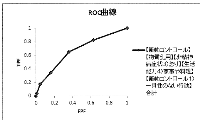
図 27 【衝動コントロール】 【物質乱用】 【非精神病症状 3) 怒り】 【生活能力 4) 家事や料理】 【衝動コントロール 1) 一貫性のない行動】 の 5 項目合計による 2 年追跡した事例の問題行動予測の ROC 曲線
