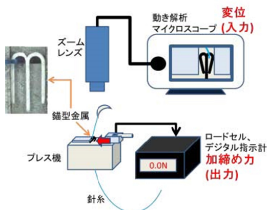
図 実験装置概要
