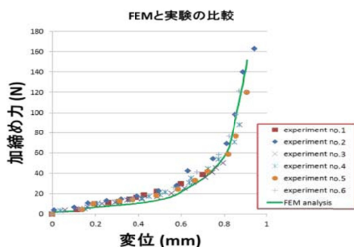
図 変位と加締め力の関係
