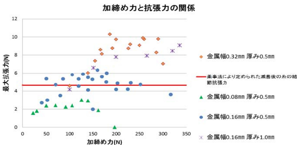
図 かしめ力と抗張力の関係
