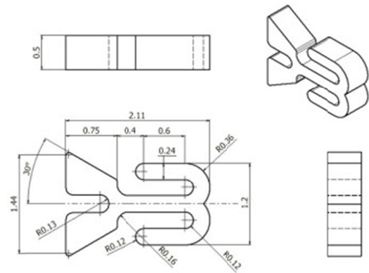
図 デバイス2の寸法
