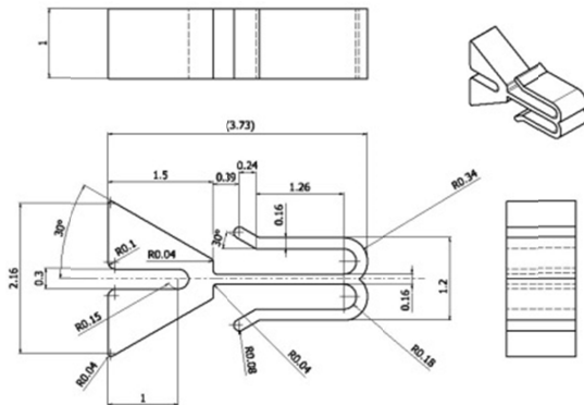
図 デバイス1の寸法
