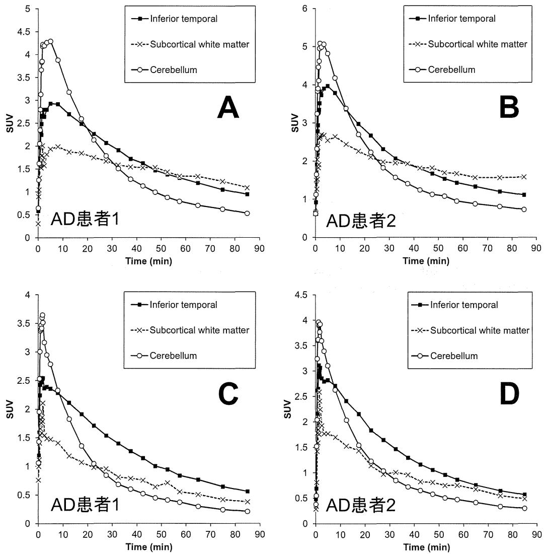
図 10 2名のアルツハイマー病患者における [^{18}\text{F}]\text{THK-5117} (A, B)、 [^{18}\text{F}]\text{THK-5351} (C, D) 投与後の時間放射能曲線の比較 (■は下部側頭葉 (Inferior temporal)、○は小脳 (Cerebellum)、×は皮質下白質 (Subcortical white matter) における時間放射能曲線を表す)
