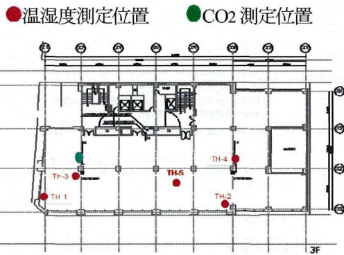
図 3-1 Tビル代表階平面図
