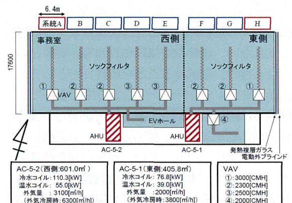
図 3-4 基準階空調設備概要
