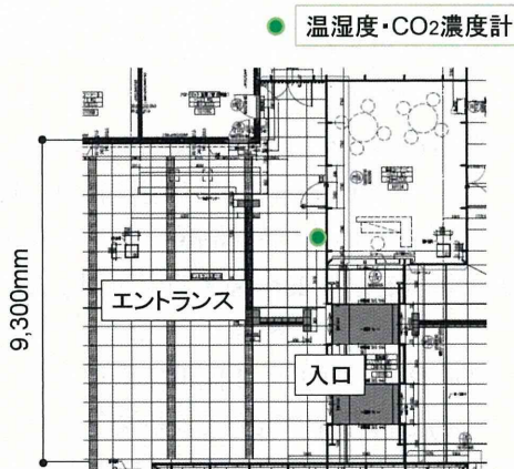
図3-11 1号館エントランス平面図
