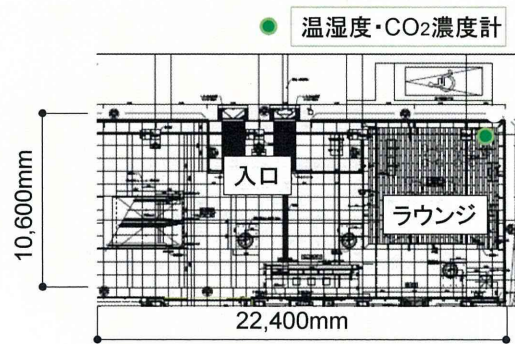
図3-13 2号館ラウンジ平面図
